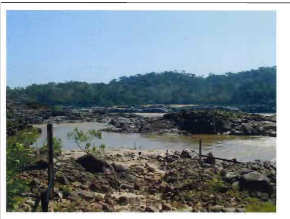
7.) La base del hidrógrama en Jirau comienza con el marco cero en el fondo del río.
