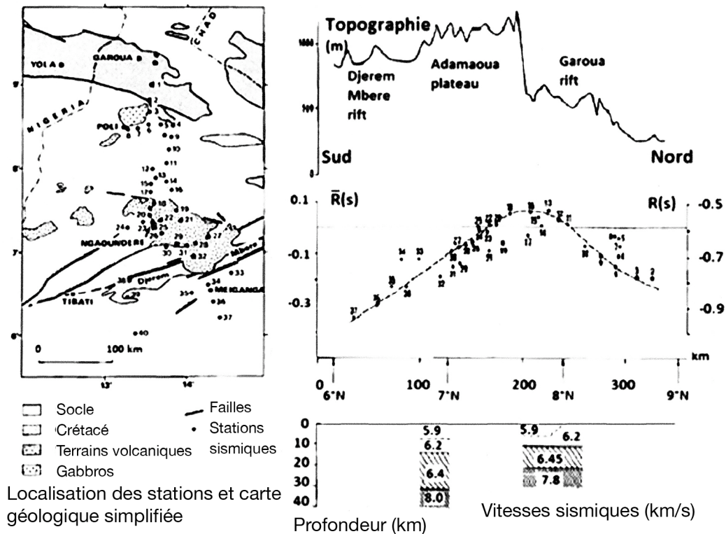
\bar{R} Résidus relatifs moyens et R résidus absolus calibrés (échelle de droite) sur une section Sud-Nord du réseau. Topographie et structure crustale interprétée
