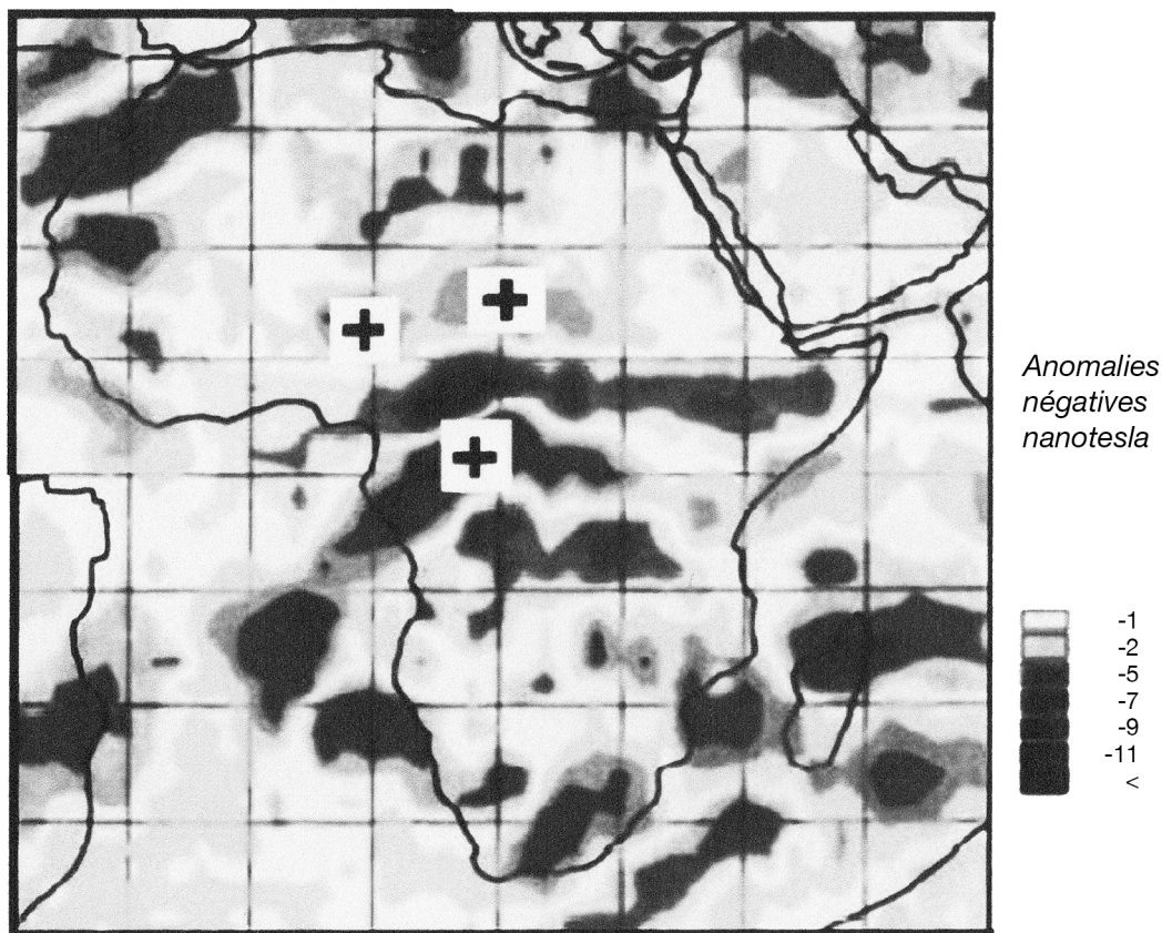
Fig. 2. Anomalies magnétiques mesurées par le satellite magsat. Les anomalies notées + sont positives.
