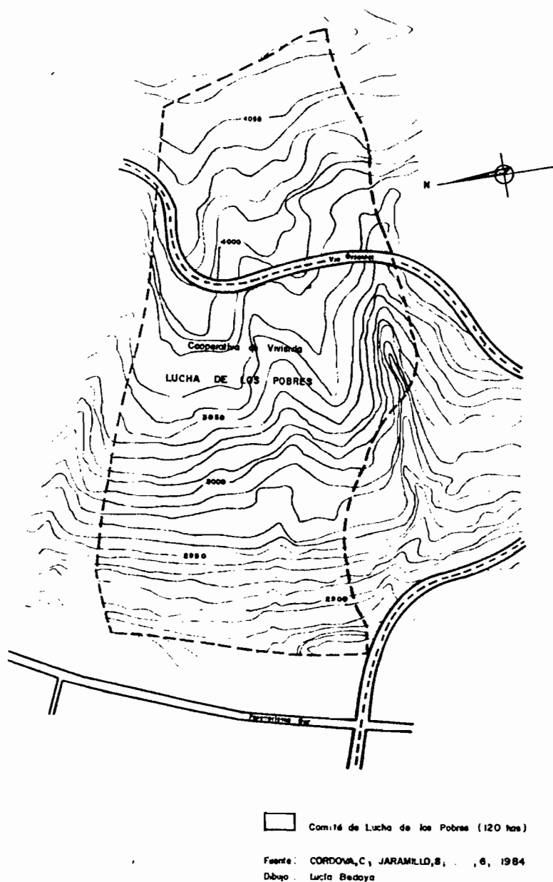
FIGURA 5 LOCALIZACION Y LIMITACIONES TOPOGRAFICAS DEL COMITE DE LUCHA DE LOS POBRES
