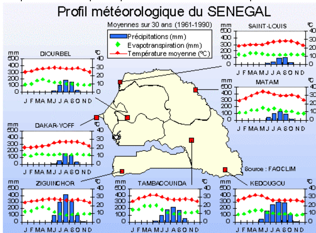
Figure 3.1 Profil météorologique du Sénégal
