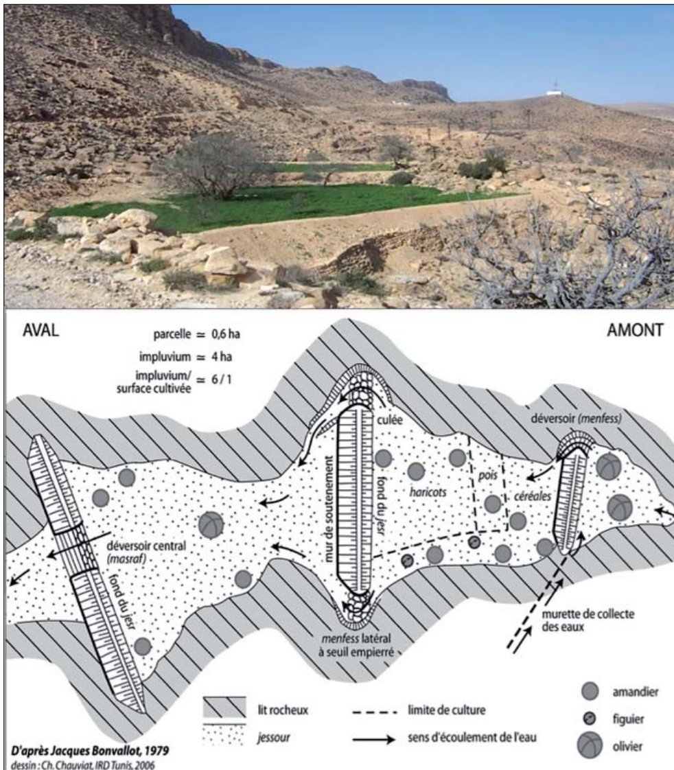
Photo 6: Schémas de fonctionnement des jessour (©IRD/B.Romagny).
