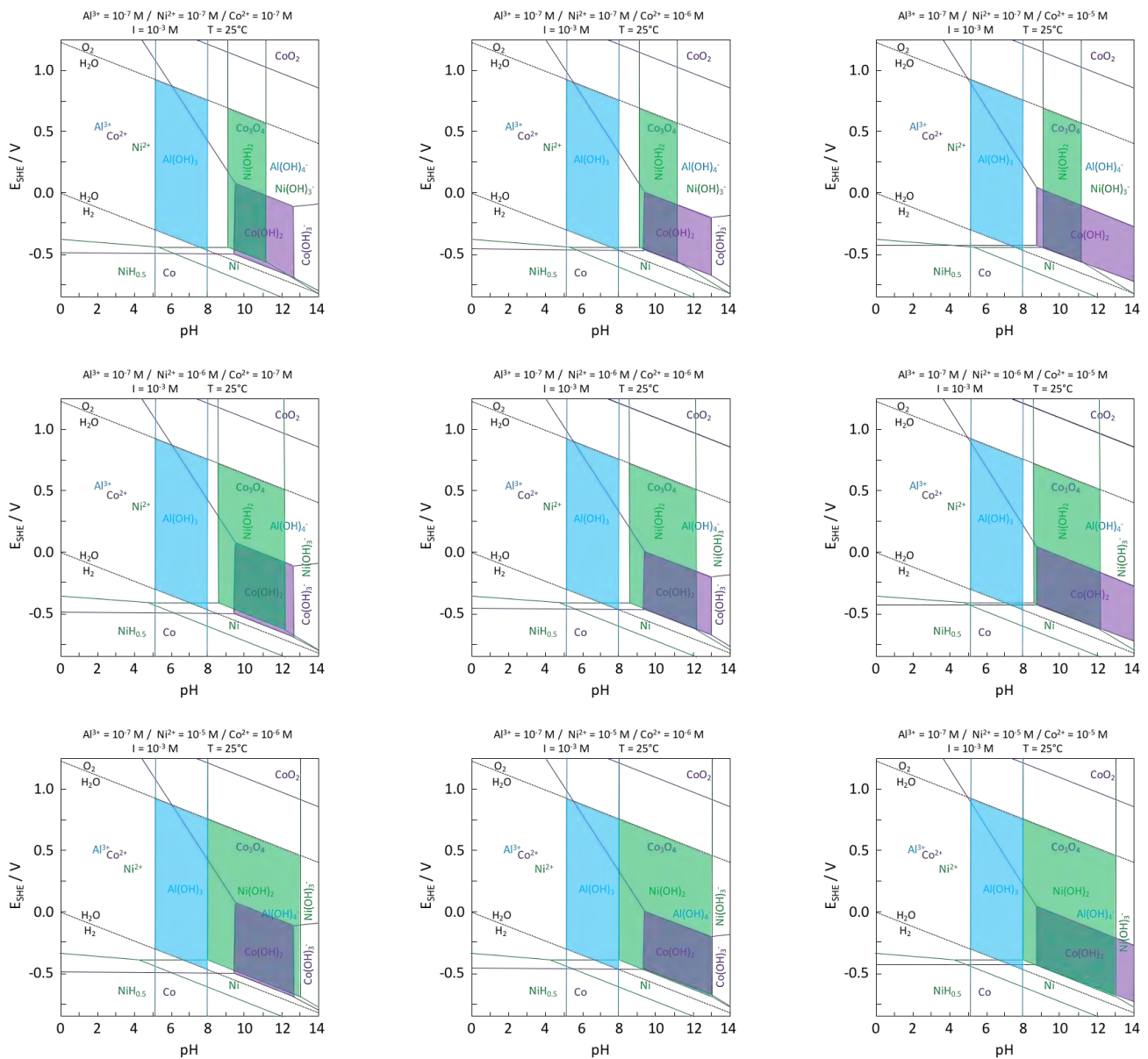
Figure 32 : Superposition des diagrammes de Pourbaix ( P_{atm} , 25°C) illustrant les zones de recouvrement éventuel des domaines de stabilité de Al(OH)_3 , Ni(OH)_2 et Co(OH)_2 (feuillet élémentaire des interstratifiés asbolane/lithiophorite du site de Goro) pour différentes concentrations en ions Ni^{2+} et Co^{2+} en solution ( [Al^{3+}] = 10^{-7} mol/L). Pour des raisons de clarté, le diagramme de Pourbaix de MnO_2 n'est pas représenté.
