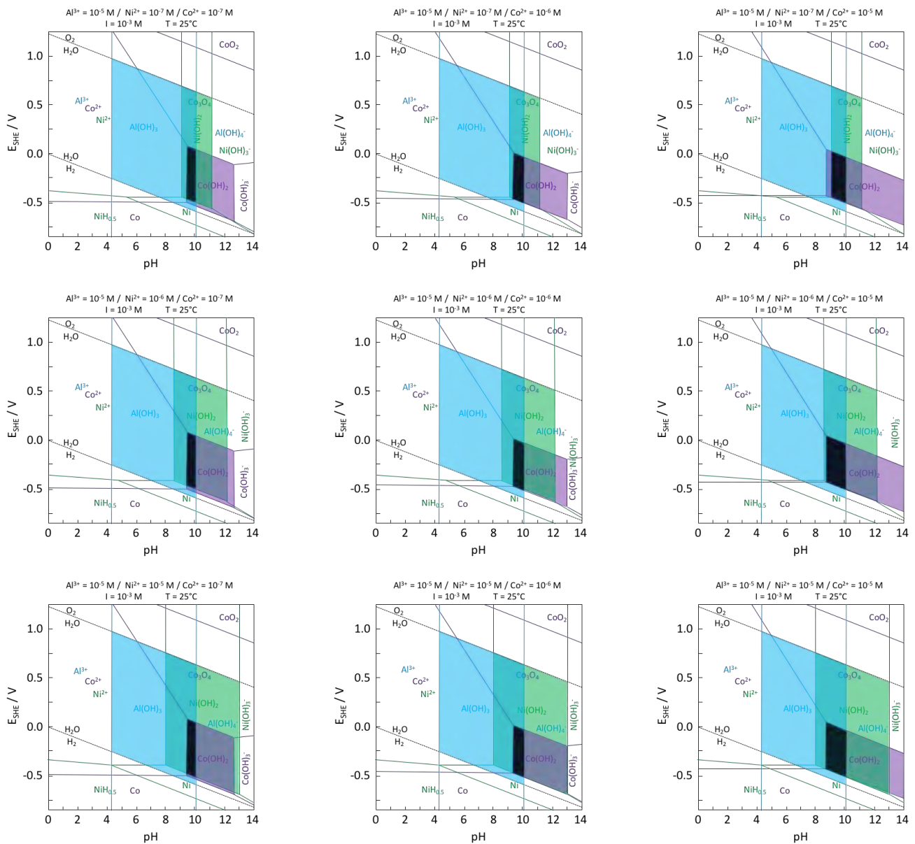
Figure 34 : Superposition des diagrammes de Pourbaix ( P_{atm} , 25°C) illustrant les zones de recouvrement éventuel des domaines de stabilité de Al(OH)_3 , Ni(OH)_2 et Co(OH)_2 (feuillets élémentaires des interstratifiés asbolane/lithiophorite du site de Goro) pour différentes concentrations en ions Ni^{2+} et Co^{2+} en solution ( [Al^{3+}] = 10^{-5} mol/L). Pour des raisons de clarté, le diagramme de Pourbaix de MnO_2 n'est pas représenté.
