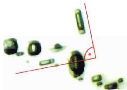
Fig. 20 - Inclusions allongées montrant deux orientations se croisant à 90°. Diascopie, 400x. Photo Gemtechlab. Elongated inclusions with two principal orientations at right angle. Diascopy, 400x.
