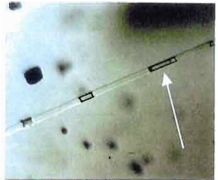
Fig. 23 - Dans un même échantillon et à température égale, le rapport des volumes occupés par les deux phases du CO 2 n'est pas constant. Si, souvent, la phase gazeuse forme de petites libelles représentant de 3 à 5% du volume de la phase liquide, certains canaux comme celui-ci présentent un rapport des deux phases plus ou moins égal à 1. De gauche à droite: Solide - H 2 O - solides - H 2 O - CO 2 liquide - H 2 O - CO 2 liquide avec une grande libelle de CO 2 gazeux (flèche) - H 2 O - CO 2 liquide. Dimensions du canal: Ø 7 µm / L 263 µm. Diascopie, lumière polarisée (//), 400x. Photo Gemtechlab.
