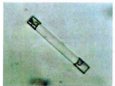
Fig. 24 - Cavité allongée et plate contenant de gauche à droite: quatre solides dans du CO 2 liquide - H 2 O - CO 2 liquide avec libelle de CO 2 gazeux. Dimensions: 9 µm / 96 µm. Diascopie, lumière polarisée (⊙), 500x. Photo Gemtechlab.
