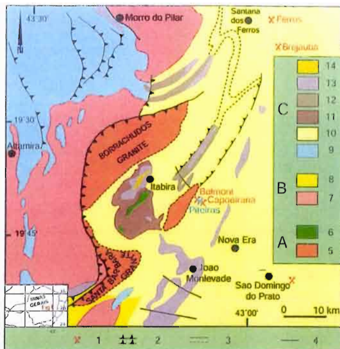
Fig. 3 - Esquisse géologique de la bordure sud ouest du craton de São Francisco et localisation des gisements et indices à émeraude du Quadrilátero Ferrífero, modifié d'après Schorsch et al., (1982). 1 : gisement et indice à émeraude ; 2 : faille de chevauchement ; 3 : contact géologique ; 4 : faille ; A : roches ultrabasiques métamorphosées et roches cataclastiques avec 5 : roches granitiques type Borrachudos, 6 : roches méla-ultrabasiques ; B : Groupe du Pré-Minas avec 7 : socle archéen, 8 : Super groupe Rio das Velhas, C : Super groupe Minas avec 9 : quartzite Espinhaço, 10 : Séquence des paragneiss, 11 : Séquence des schistes verts, 12 : Groupe Caraça, 13 : Groupe Itabira, 14 : Groupe Piracicaba. Geological sketch of the southwestern border of the São Francisco craton with the location of the deposits and occurrences of emerald in the Quadrilátero Ferrífero, modified from Schorsch et al., (1982). 1 : deposit and occurrence of emerald, 2 : thrust fault, 3 : geological contact, 4 : fault, A : meta-ultrabasic and cataclastic rocks with 5 : granitic rocks type Borrachudos, 6 : meta-ultrabasics ; B : Pre-Minas Group with 7 : Archean basement, 8 : Rio das Velhas Super Group, C : Minas Super Group with 9 : Espinhaço quartzite, 10 : paragneiss sequence, 11 : green schist sequence, 12 : Caraça Group, 13 : Itabira Group, 14 : Piracicaba Group.
