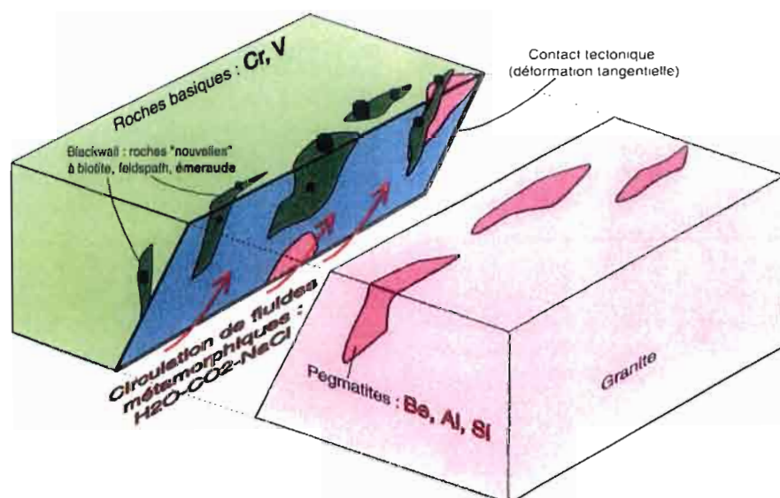
Fig. 12 - Schéma génétique proposé pour la formation des émeraude de Piteiras-Capoeirana-Belmont. Les fluides hydrothermaux, d'origine métamorphique (flèches rouges), circulèrent durant l'orogénèse Brasiliano (il y a 508 millions d'années) suivant le plan de contact (zone tectonique majeure de la région) entre des granites déformés (dont les pegmatites contiennent du béryllium) et des roches basiques (riches en chrome et vanadium). Les fluides en réagissant avec les deux roches mettent en solution tous les éléments chimiques nécessaires à la cristallisation de l'émeraude (Be, Al [Cr, V, Mg, Fe, Na, H 2 O, etc.], Si, O). Le résultat final de cette interaction fluide-roche est la production de nouvelles roches qui peuvent contenir l'émeraude à savoir des feldspathites (anciennes pegmatites dont le quartz a été dissous et remplacé par du feldspath) et des schistes à phlogopite (l'équivalent du blackwall ou des schistes à phlogopite ou des phlogopitites de certains auteurs) qui se sont formés à l'insu des roches basiques.
