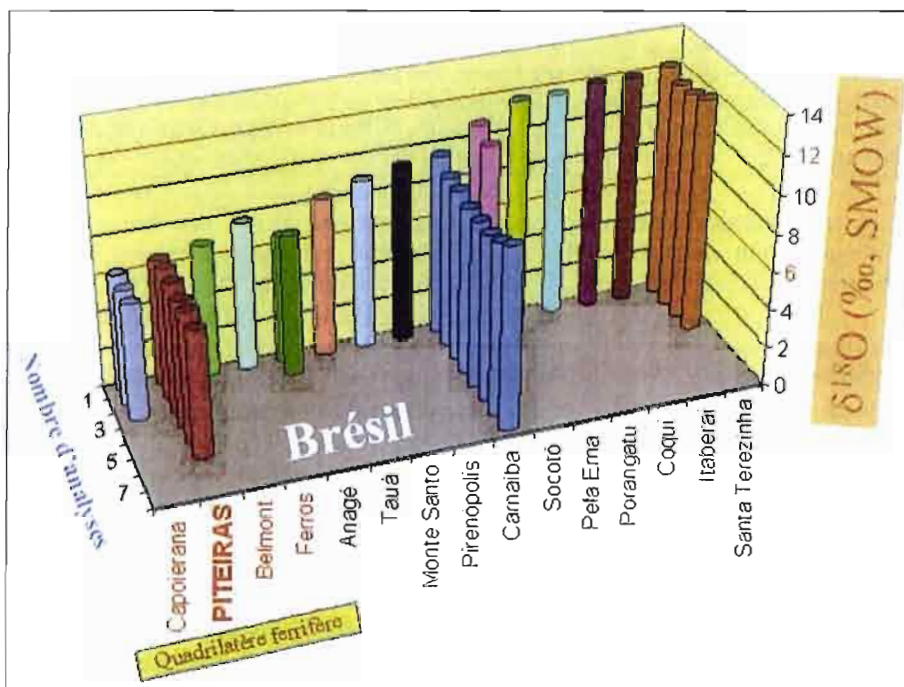
Fig. 8 - Histogramme des rapports isotopiques de l'oxygène des émeraudes brésiliennes ( \delta^{18}\text{O} , ‰ par rapport au SMOW). Les valeurs isotopiques obtenues pour les émeraudes de Capoeirana, Piteiras et Belmont sont les plus légères au monde.
