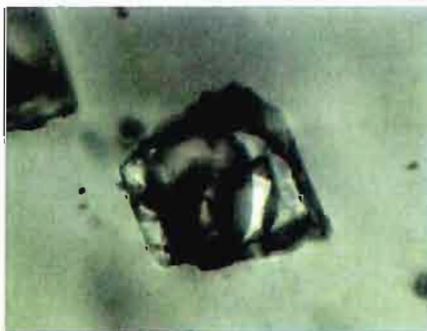
Fig. 19 - Cavité contenant H 2 O, CO 2 liquide, CO 2 gazeux et un solide qui malgré sa ressemblance apparente avec du quartz est un feldspath. Lumière polarisée (//). 500x. Photo Gemtechlab.
