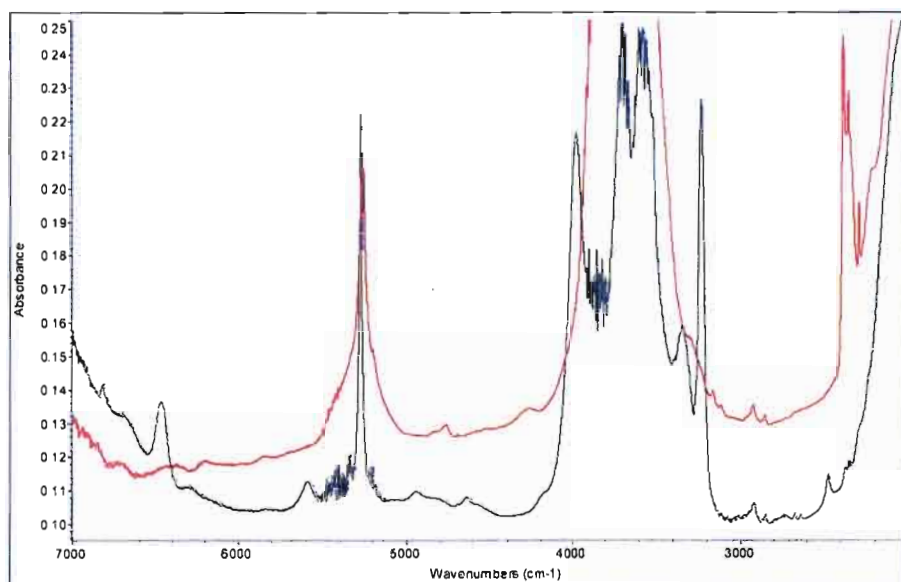
Fig. 37 - Spectre infrarouge polarisé d'une émeraude de Piteiras (faisceau \perp "c"). En rouge : rayon extraordinaire, en bleu : rayon ordinaire
