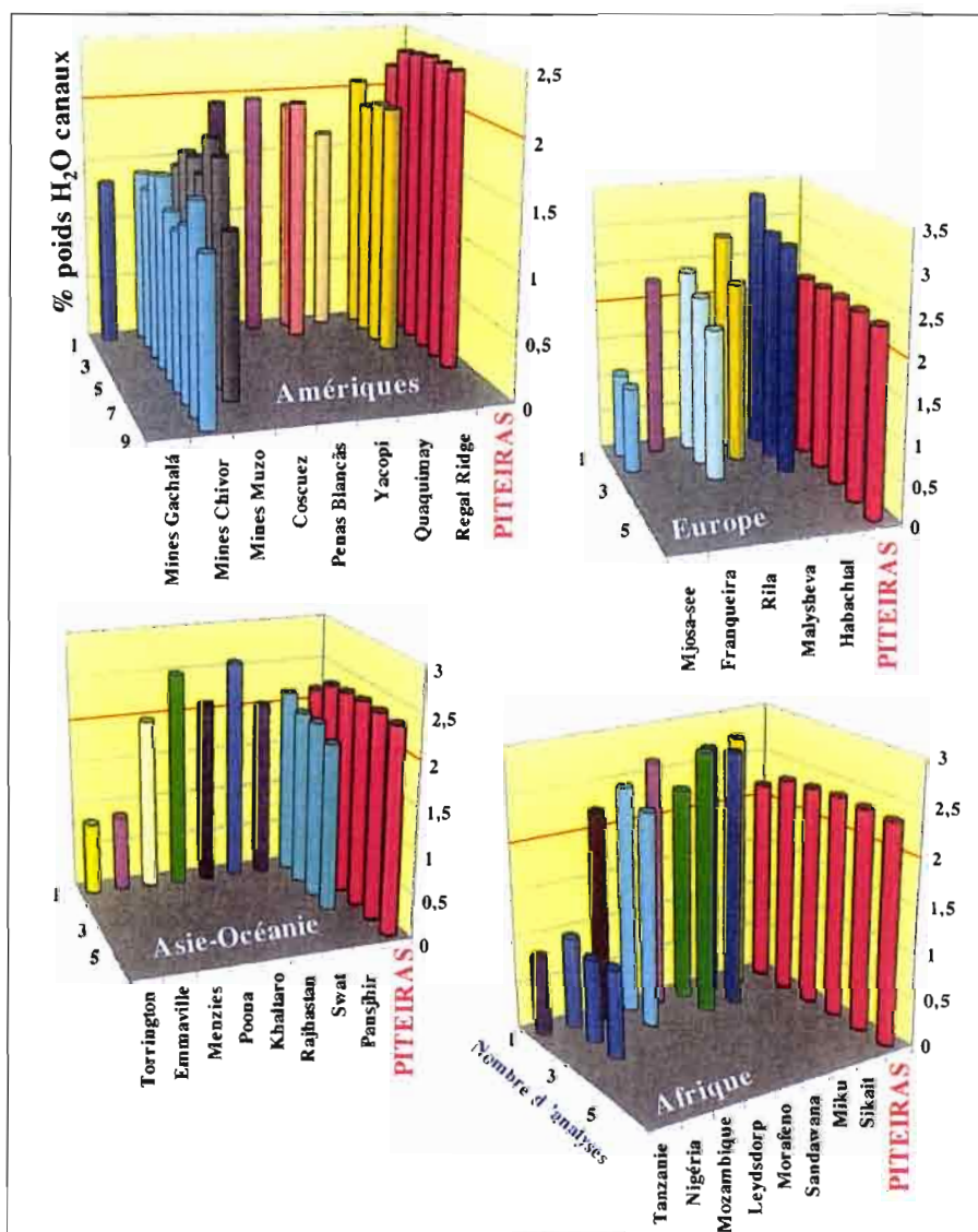
Fig. 11 - Histogramme de la quantite d'eau contenue dans la plupart des émeraude connues au monde. Dans chaque histogramme, les émeraude de Piteiras sont reportées en référence. Le détail des données est précisé dans Groal et al., (2002) Histogram of channel water content for different emeralds worldwide. For each histogram, the Piteiras emeralds are reported for comparison. The data are detailed in Groal et al., (2002).
