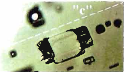
Fig. 32 - Cristal d'albite prolongé (à droite) par une cavité contenant du CO 2 liquide. La longueur apparente de l'albite est parallèle à l'axe "c" de l'émeraude. Diascopie, lumière polarisée (⊗), 400x. Photo Gemteclab.
