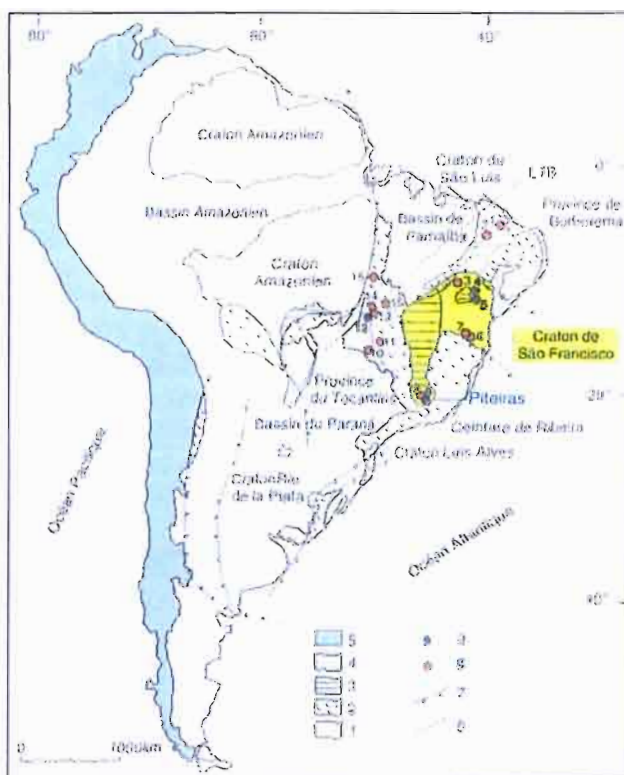
Fig 1 - Le Précambrien dans le continent Sud-Américain (localisation des différents indices et mines d'émeraude, modifié d'après Brito Neves et Cordani, 1991)
