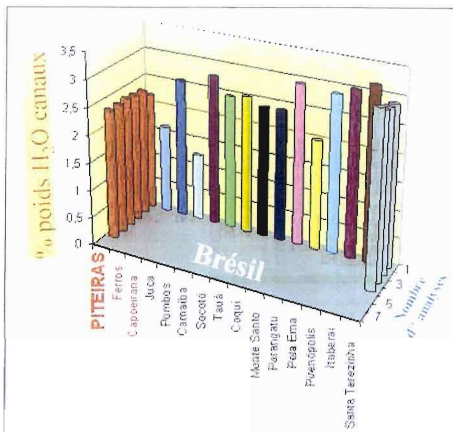
Fig. 10 - Histogramme de la quantité d'eau contenue dans les émeraudes du Brésil (en % poids). La quantité d'eau contenue dans les inclusions fluides observables sous le microscope est négligeable. Elle représente à peu près 0,1 % poids de la quantité totale de l'eau totale contenue dans une émeraude. Pour toutes nos expériences, cette eau a été préalablement éliminée par décrépitation, à 550°C, des inclusions fluides.
