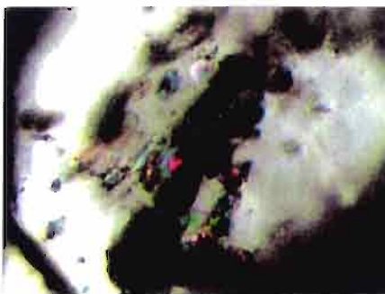
Fig. 34 - Inclusions du même cristal d'albite. Diascopie, immersion, lumière polarisée (⊗), 100x. Photo Gemteclab.
