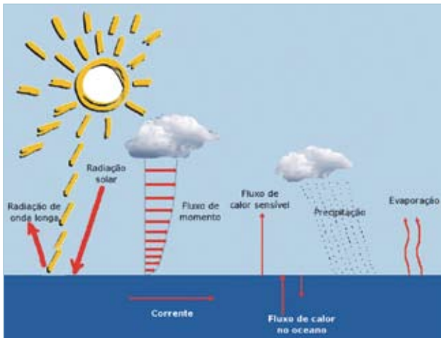
Figura 9. Esquema representativo dos fluxos verticais de energia, massa e quantidade de movimento entre a atmosfera e o mar. Esses fluxos verticais serão mostrados no ASPSP pelo Projeto FluTuA.
