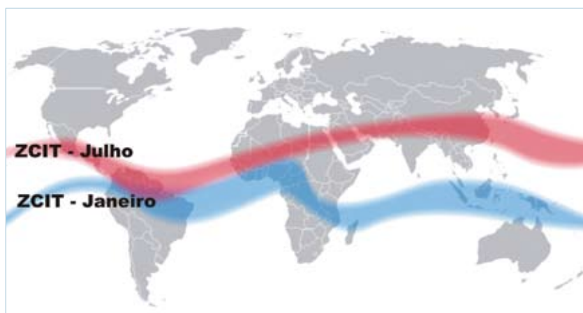
Figura 4. Posição média da zona de convergência intertropical (ZCIT) em julho (vermelho) e janeiro (azul).
