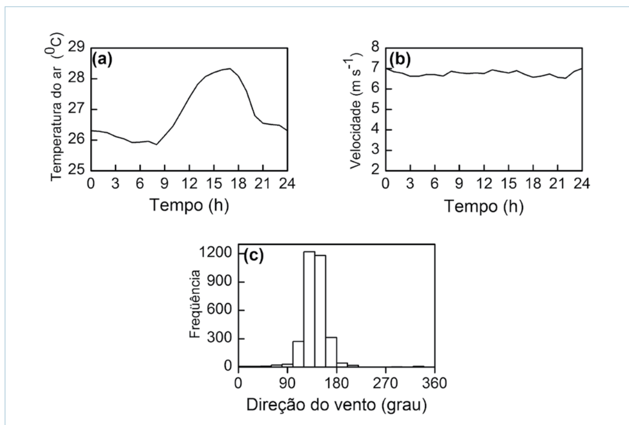
Figura 7. Dados da estação meteorológica automática mantida pelo Instituto Nacional de Meteorologia (INMET) no ASPSP e representativos do microclima da ilha Belmonte. (a) Temperatura do ar ( ^{\circ}\text{C} ) em função da hora do dia; (b) velocidade do vento ( \text{m s}^{-1} ) em função da hora do dia e (c) histograma da direção do vento.
