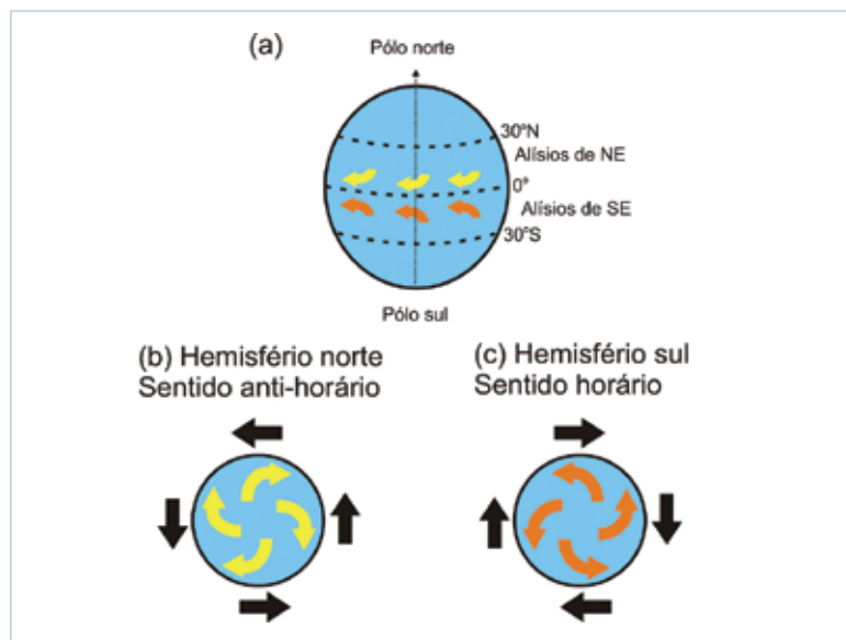
Figura 3. Representação esquemática (a) dos ventos alísios na faixa equatorial da Terra e do sentido de rotação da Terra nos hemisférios (b) norte e (c) sul. As setas internas ao globo terrestre indicam a deflexão sofrida pelos ventos próximos à superfície. As setas externas ao globo indicam o sentido de rotação da Terra vista do respectivo pólo.
