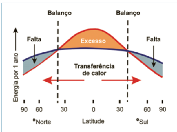
Figura 2. Esquema da distribuição do saldo de energia, por ano, em função da latitude. Figure 2. Diagram of the energy net distribution, per year, in function of the latitude.
