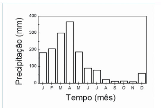
Figura 5. Precipitação observada (mm) em função dos meses do ano. Dados obtidos pela bóia 0° N-35° W do Programa PIRATA.
