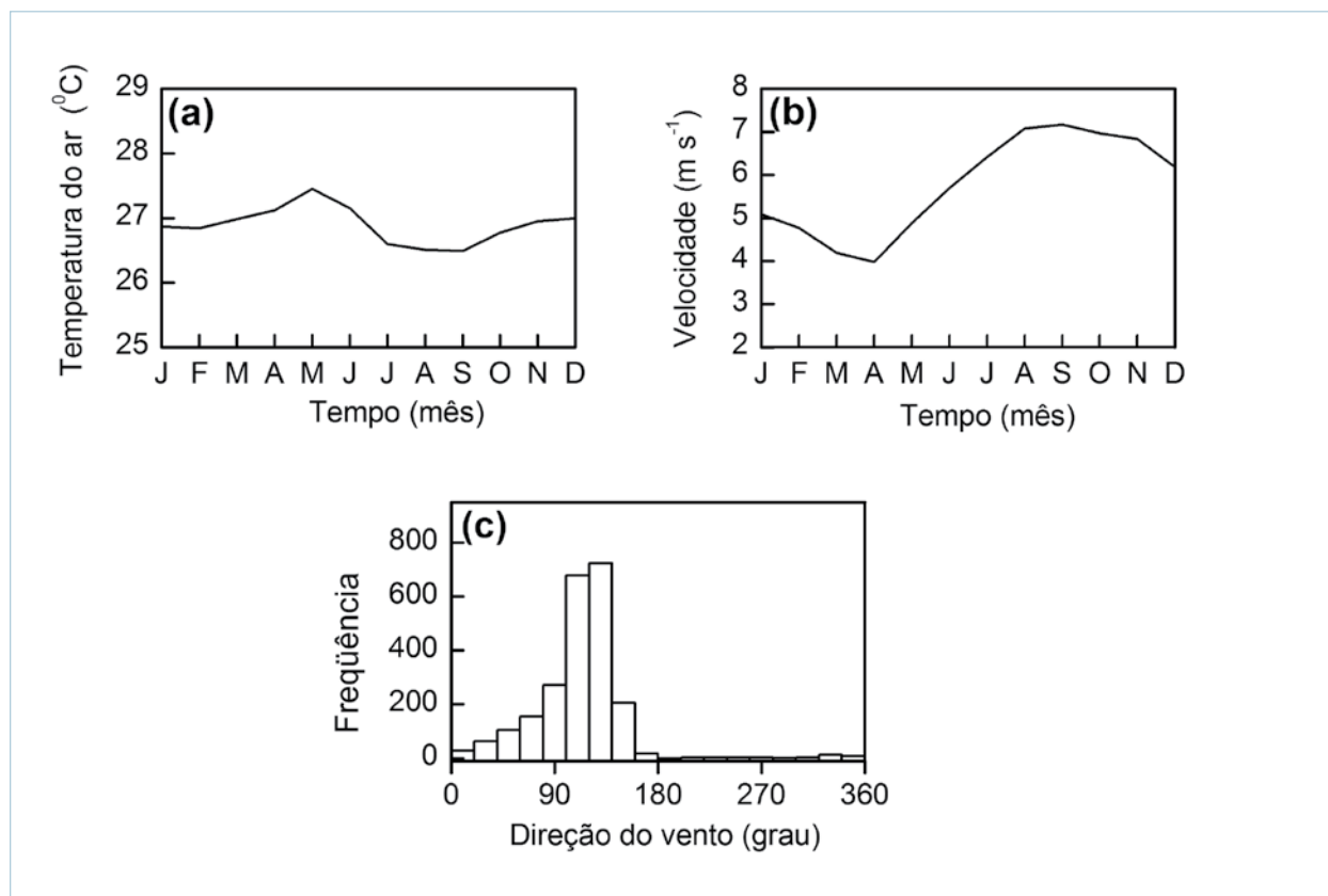
Figura 8. Dados obtidos pela bóia PIRATA localizada em 0^{\circ}\text{N} - 35^{\circ}\text{W} . (a) Temperatura do ar ( ^{\circ}\text{C} ) em função dos meses do ano; (b) velocidade do vento ( \text{m s}^{-1} ) em função dos meses do ano; e (c) histograma da direção do vento.
