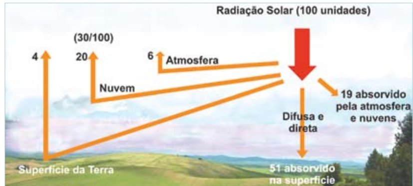
Figura 1. Esquema do balanço global de radiação no sistema Terra-atmosfera. Figure 1. Diagram of the global balance of radiation in the Earth-atmosphere system.
