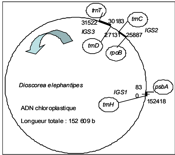
Figures 3. 3a -Position des six gènes encadrants les trois espaces intergéniques sélectionnés (IGS) sur la carte du génome chloroplastique de Dioscorea (HANSEN, et al. 2007). 3b-Exemple de séquence consensus (IGS1 de D. villosa ).
