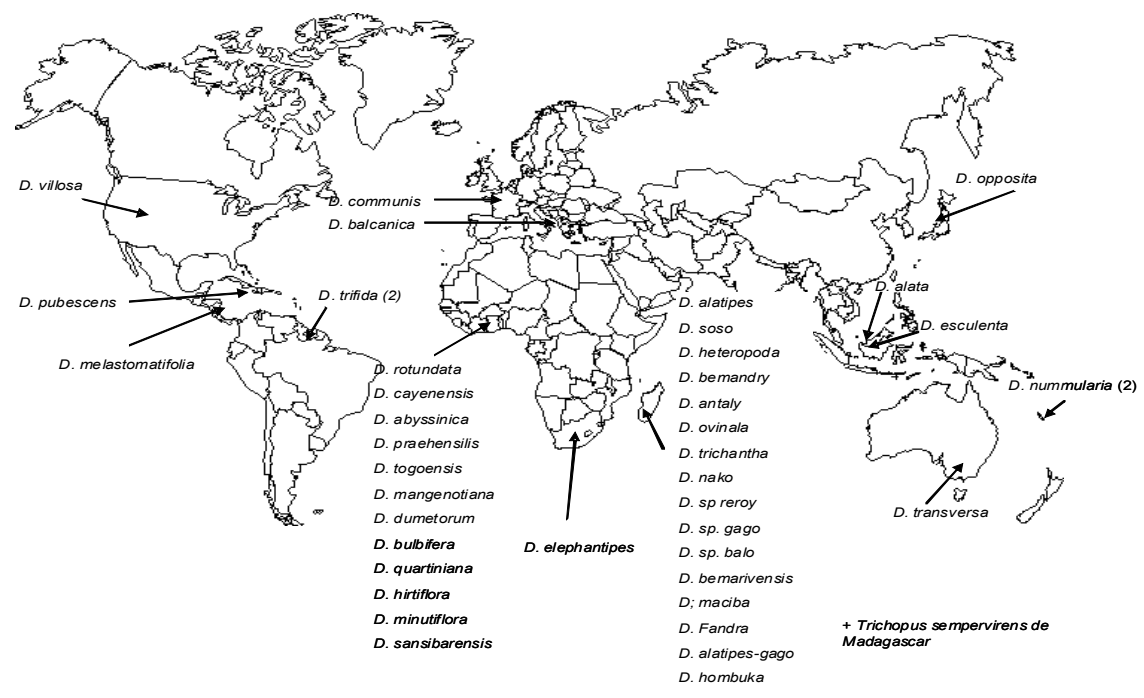
Figure 2 : Répartition géographique des espèces étudiées.
