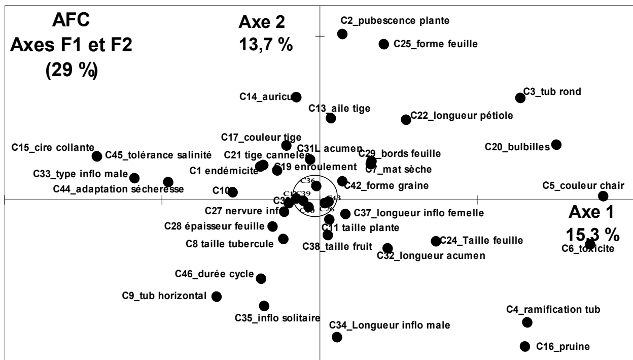
Figures 7a : Axes 1 et 2 (29% de la diversité observée) d'une analyse factorielle des correspondances (AFC) des 24 espèces du Sud de Madagascar et de 46 caractères morphologiques.
