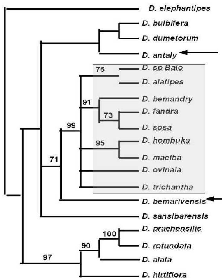
Figure 5 : Arbre phylogénétique de parcimonie stricte des séquences consensus de trois IGS chloroplastiques de 19 espèces (onzes malgaches du Sud sans D. nako ). D. elephantipes est utilisée comme élément externe. Sur les branches, les valeurs de bootstraps ont été signalées. L'encadré signale un important groupe d'ignames endémiques. Les flèches signalent les deux espèces endémiques différentes des autres.
