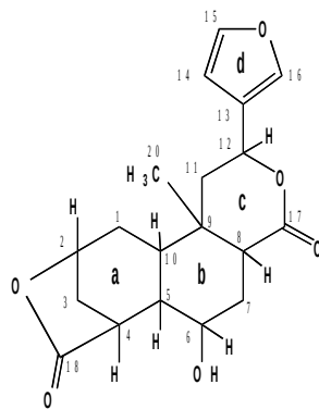
8-épi-diosbulbine E
