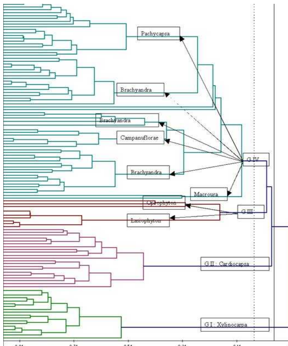
Figure 8 : Classification ascendante hiérarchique, CAH, des 119 plantes de 14 espèces (logiciel XLSTAT).
