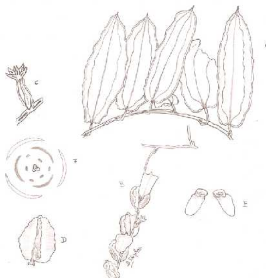
Figures 3 : Dioscorea sp. ( reroy ou rerohy ). Partie végétative et morphologie florale femelle. A : Feuilles pétioles avec trois nervures et un petit acumen ; B : Fruits et inflorescence femelle en grappe ; C : Fleur femelle vue de profil ; D : Capsule immature avec bractée ; E : Graines avec une grande aile ; F : Diagramme floral de la fleur femelle. A : Planche d'herbier SD 364 ; B, D : Planche d'herbier SD 109 ; C, E, F : Planche d'herbier SD 115.
