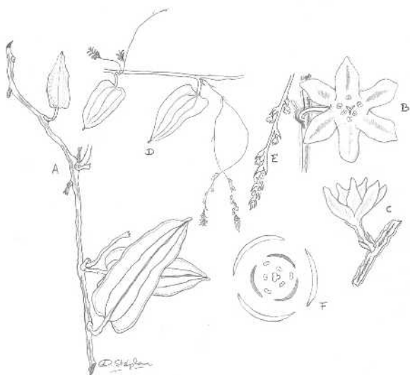
Figures 2 : Dioscorea sp. ( reroy ou rerohy ). Partie végétative et morphologie florale mâle. A : tige robuste avec feuilles pétioles et alternes ; B : Fleur mâle vue de face avec six étamines ; C : Fleur mâle vue de profil avec cuticule ; D : Inflorescence mâle pendante ; E : Inflorescence mâle en grappe ; F : Diagramme floral de la fleur mâle. B, C, et F : planche d'herbier SD 116 ; D, E : planche d'herbier SD 110.
