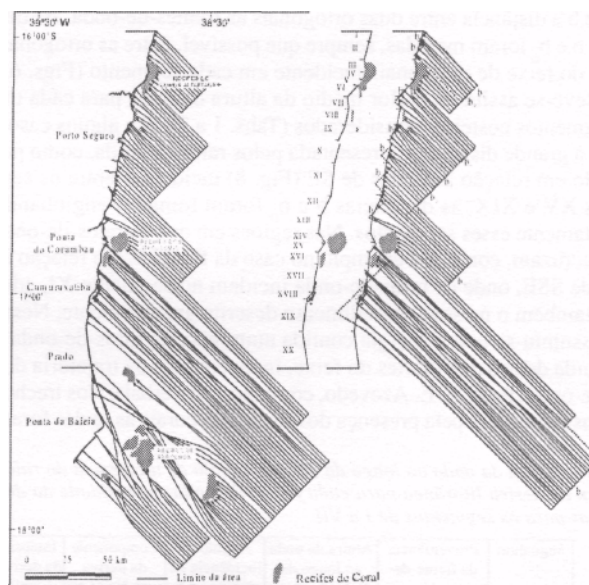
Figura 8 - Diagrama de refração para ondas provenientes de SE (N135°), com período de 6,5s (esquerda). Segmentação da linha da costa em trechos retilíneos (centro). Medidas de b e b_0 (ver texto) (direita).
