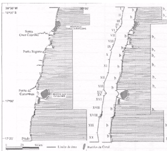
Figura 7 - Diagrama de refração para ondas provenientes de E (N90°), com período de 5s (esquerda). Segmentação da linha da costa em trechos retilíneos (centro). Medidas de b e b_0 (ver texto) (direita).
