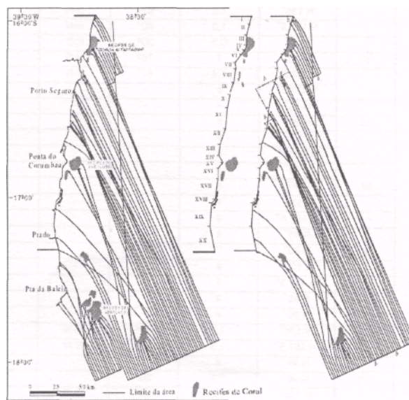
Figura 9 - Diagrama de refração para ondas provenientes de SSE (N157,5°), com período de 6,5s (esquerda). Segmentação da linha da costa em trechos retilíneos (centro). Medidas de b e b_0 (ver texto) (direita).
