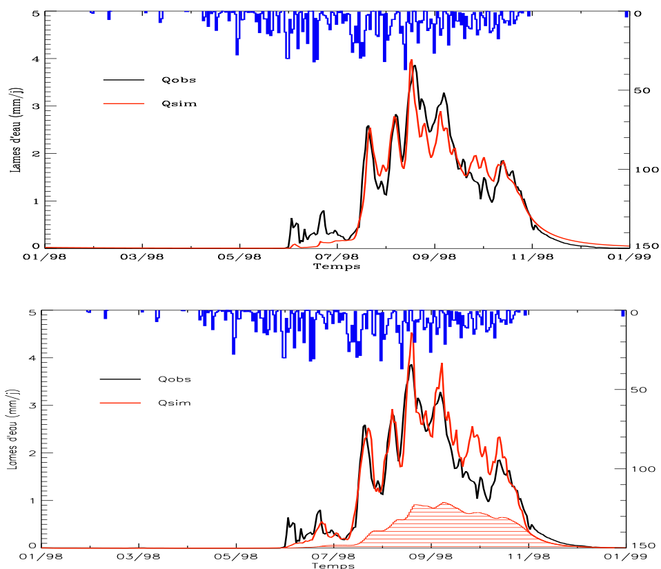
FIG. 5.6: Hyétogramme et hydrogramme de 1998 sur l'Ouébé à Bétérou. Simulations GR4J (en haut) et TOPAMMA (en bas) (calage 1998-2002)
