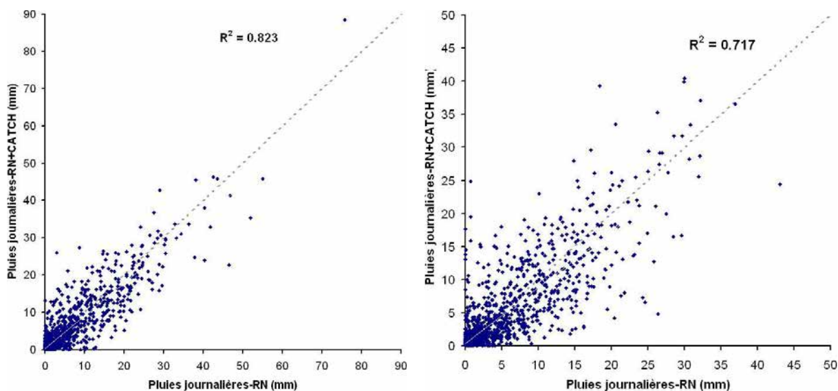
FIG. 3.8: Corrélation des lames d'eau journalières moyennes, krigées à partir du Réseau National (RN) et du réseau complet (RN+CATCH) sur les bassins de la Donga (à gauche) et de l'Ouémé à Bétérou (à droite), pour la période 1998-2002
