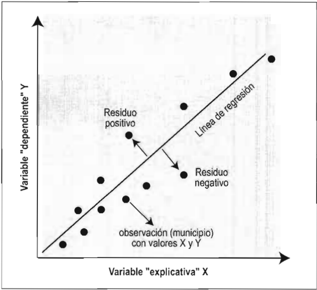
Figura 41: Gráfico de la regresión
