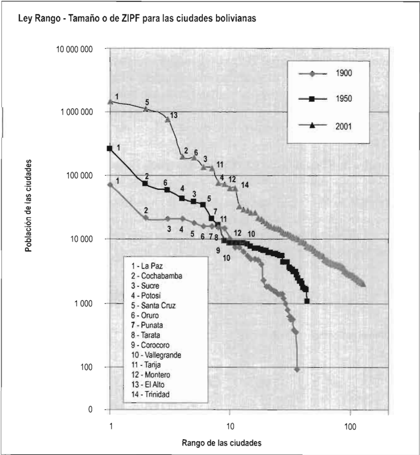
Figura 7: Gráfico de la ley rango-tamaño
