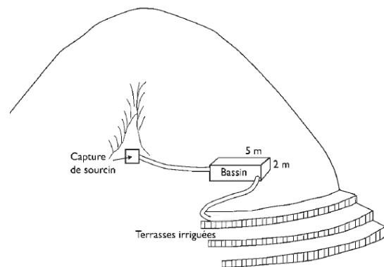
Schémas de capture et stockage des eaux de sourcins.
