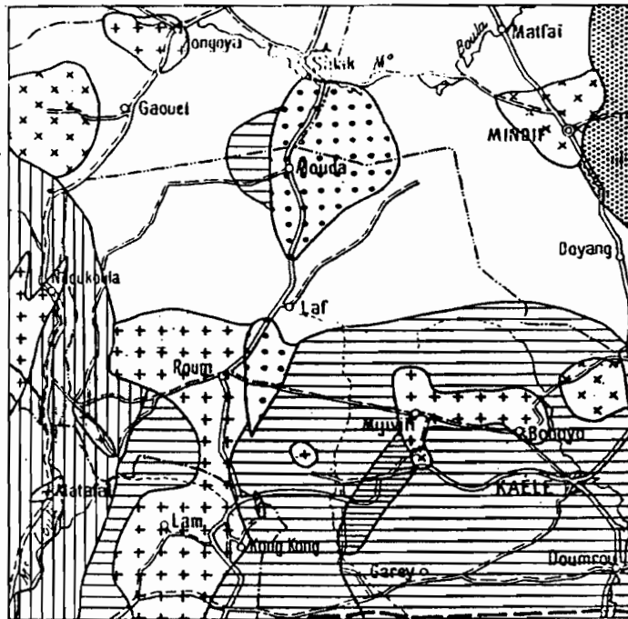
b - GÉOLOGIE
