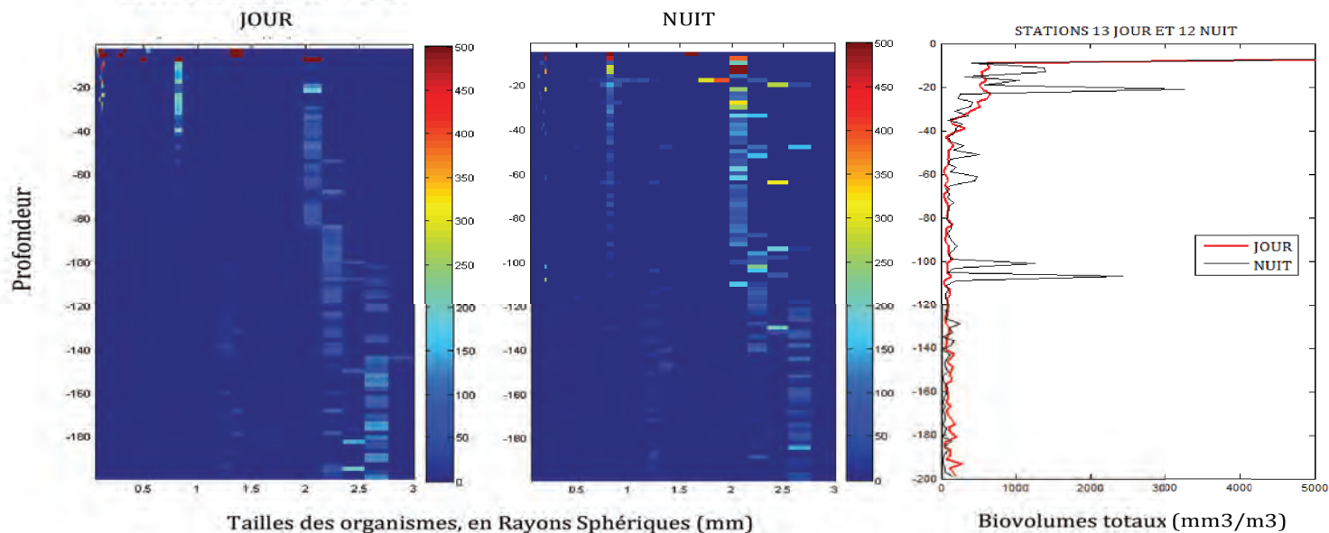
Biovolumes par classes de tailles et par profondeur ( \text{mm}^3/\text{m}^3 )
