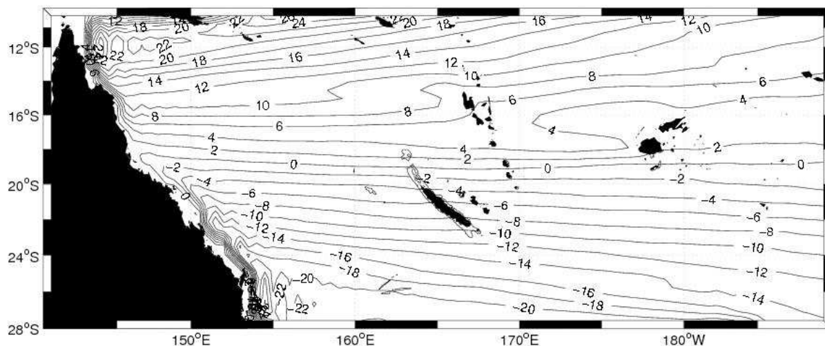
figure VI-11 : Fonction de courant barotrope obtenu avec ROMS dans sa configuration « fond plat/Linéaire » et en absence des îles ( 1/2^\circ ).
