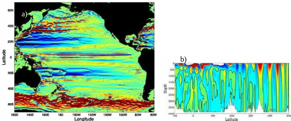
figure II-3 : a) Vitesse zonale moyenne (3 ans) à 400m issue du modèle MOM3. b) Section verticale de vitesse zonale à 180E. Les couleurs saturant à -0.06 m/s (bleu) et 0.06 m/s (rouge). D'après Richards et al. (2006)
