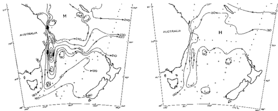
figure I-8 : Topographie géopotentielle (Hauteurs dynamique) en surface (à gauche) et à 400 db (à droite) relative à 1750db, d'après Wyrtki (1962).
