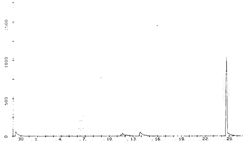
Ravine RENEVILLE à POMBIRAY - Hydrogramme des crues de mai 1988.
