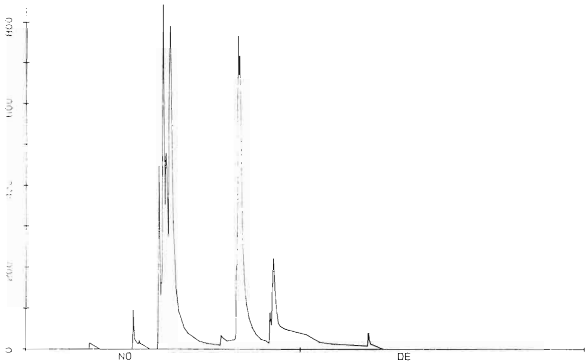
Ravine RENEVILLE à POMBIRAY - Hydrogramme des crues de novembre et décembre 1988.
