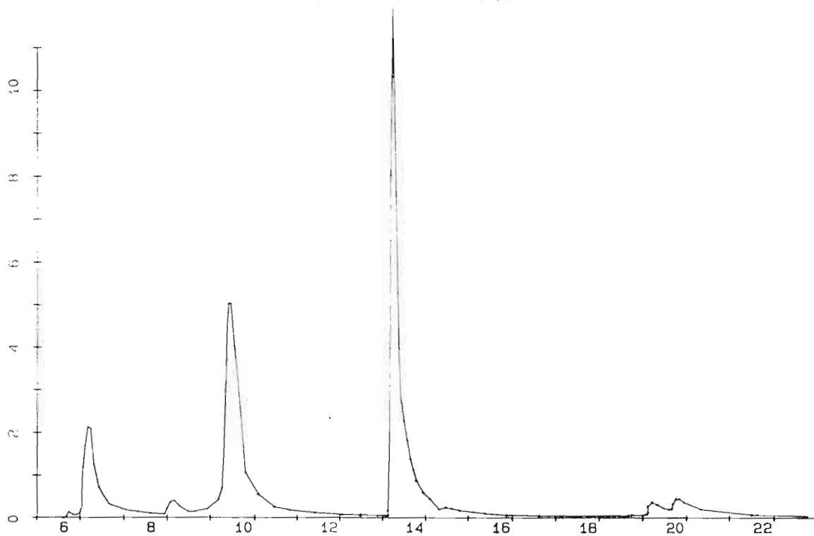
Ravine RENEVILLE à POMBIRAY - Hydrogramme des crues de septembre 1988.
