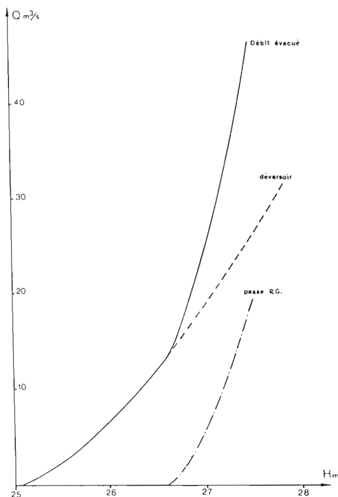
Débits évacués par les seuils.
