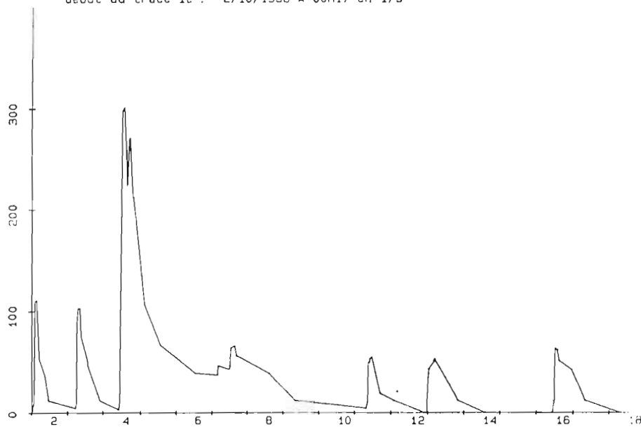
Ravine RENEVILLE à POMBIRAY - Hydrogramme des crues d'octobre 1988.
