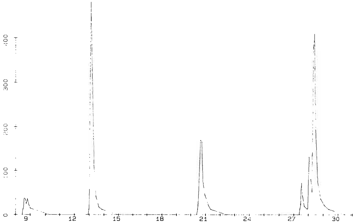
Ravine RENEVILLE à POMBIRAY - Hydrogramme des crues de juillet 1988.
