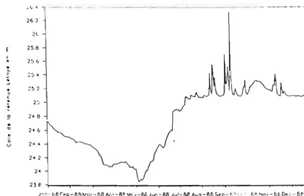
Variations journalières des cotes de la retenue.
