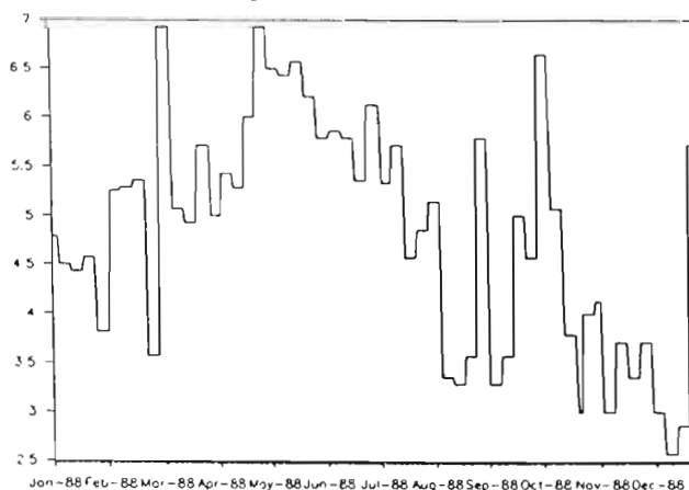
Répartition de l'évaporation journalière au cours de 1988.
