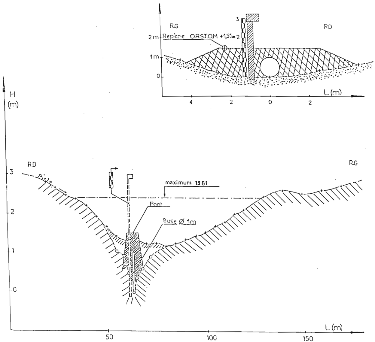
Profils en travers de la station de POMBIRAY.
