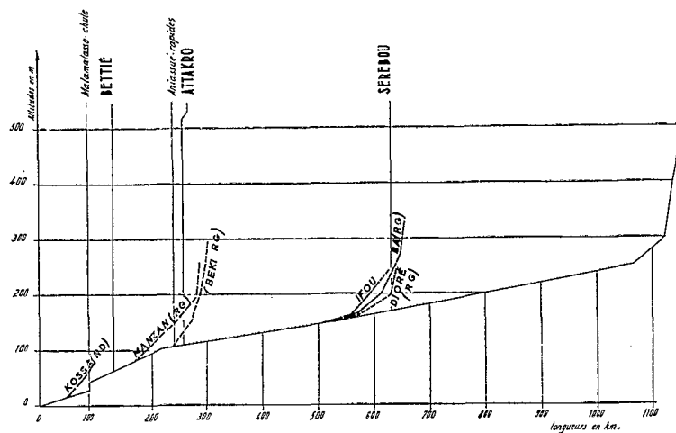
FIG. 7. — LA COMOÉ. Profil en long.
