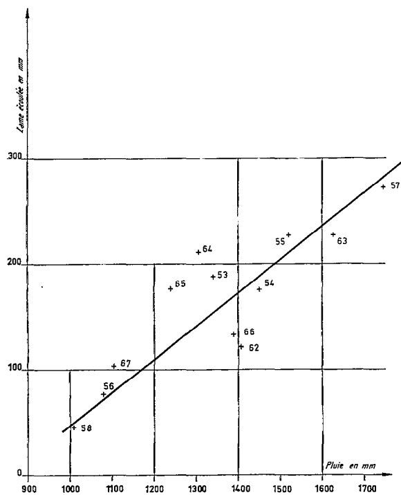
FIG. 15. — Lame écoulee annuelle en fonction de la pluie moyenne. Bassin du BANDAMA à BRIMBO.
