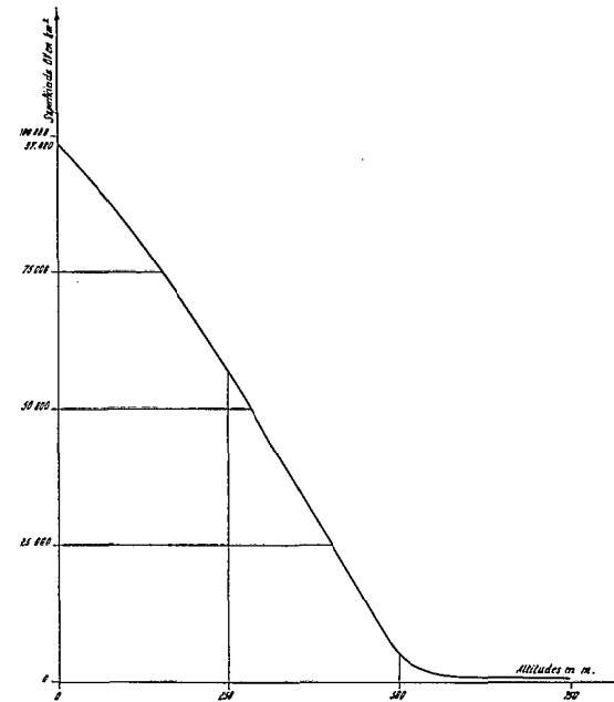
FIG. 6. — LE BANDAMA. Courbe hypsométrique.
