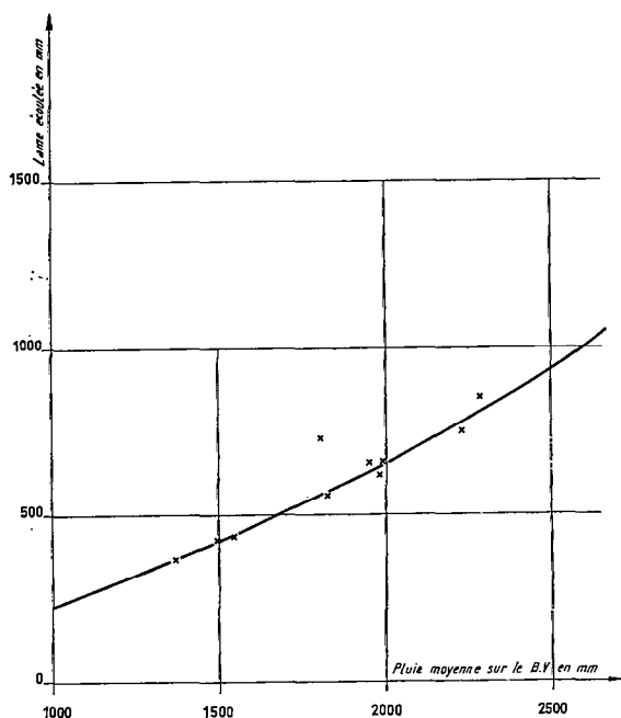
FIG. 13. — Lame écoulee annuelle en fonction de la pluie moyenne Bassin du CAVALLY à FLAMPLEU.
