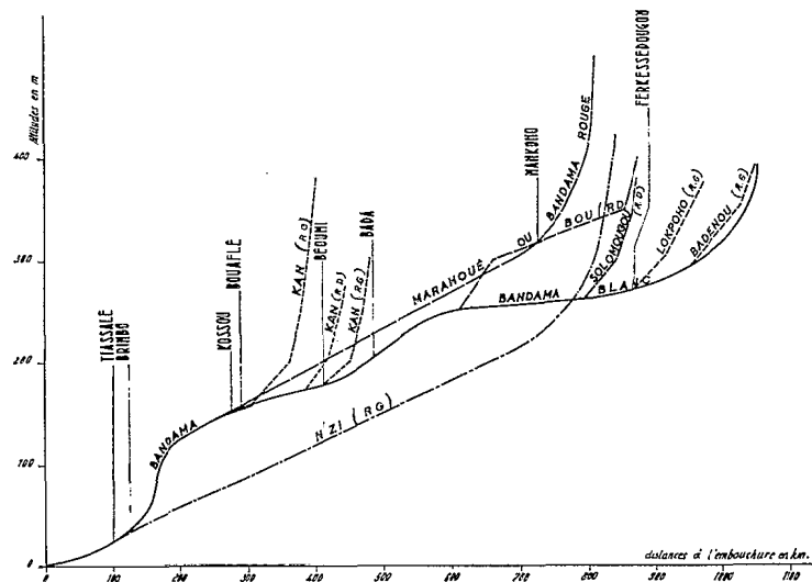
FIG. 5. — LE BANDAMA. Profil en long.
