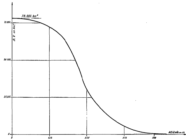
FIG. 8. — LA COMOÉ. Courbe hypsométrique.
