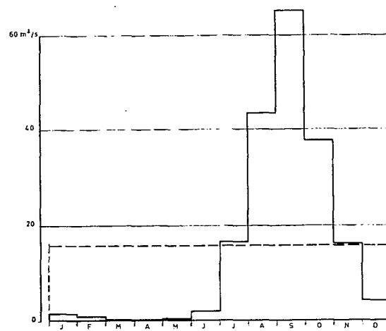
FIG. 20. — Débits moyens mensuels. La BAGOË à GUIN-GÉRINI.
