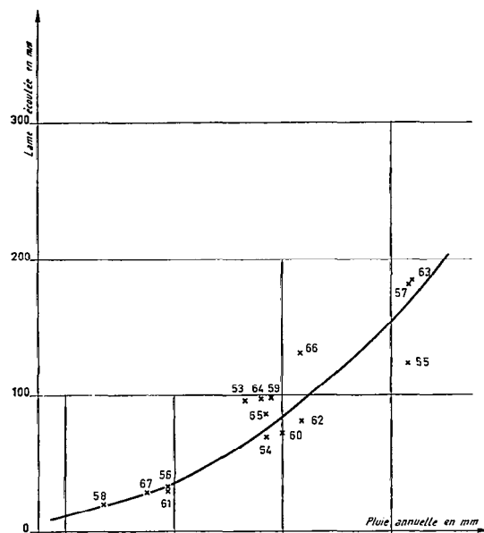
FIG. 14. — Lame écoulee annuelle en fonction de la pluie moyenne. Bassin du NZI à ZIÉNOA.
