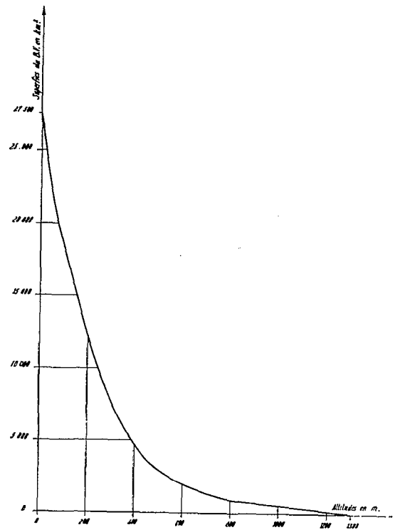
FIG. 3. — LE CAVALLY. En amont de Tiboto (Grabo). Courbe hypsométrique.
