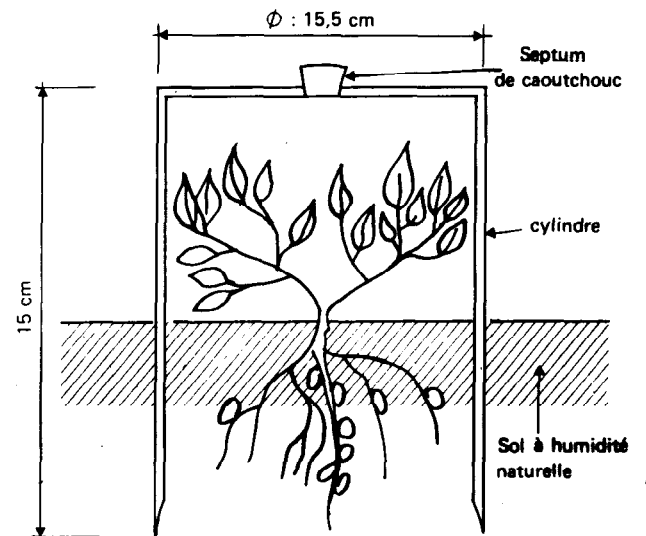
FIG. 3. - Coupe schématique du dispositif de mesure in situ de l'activité nitrogénasique (cylindre de BALANDREAU et DOMMEGUES modifié).
