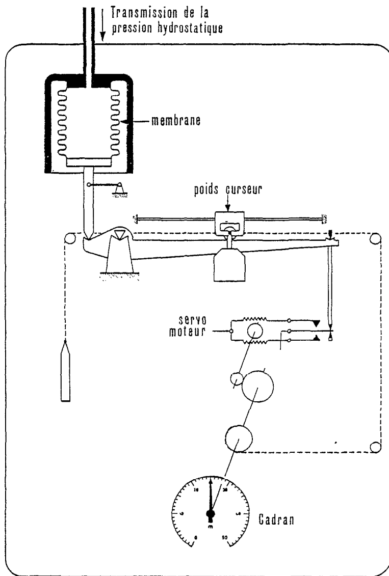
BALANCE DE PRESSION RITTMAYER . SCHEMA DE PRINCIPE .
