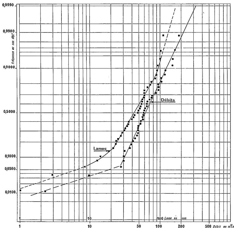
Fig. 13. — Distribution des débits journaliers maximaux annuels et des lames annuelles simulées de l'oued Ghorfa à Ouled-Addet (1 120 km 2 ) à partir de la série pluviométrique de M'Bout
