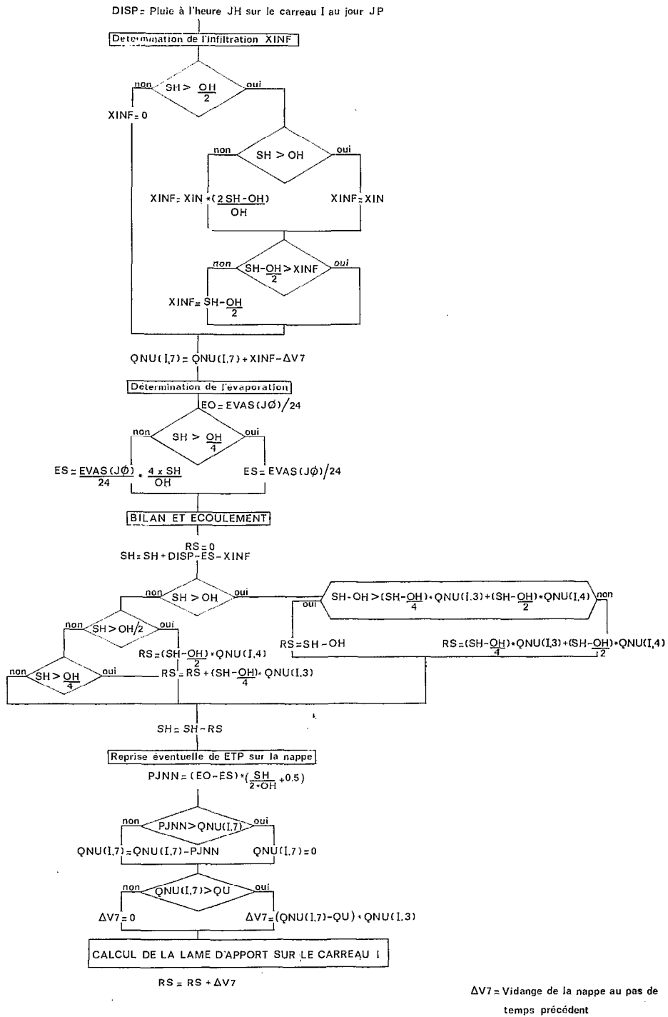
Fig. 5. — Fonction horaire de production (oued Ghorfa)
