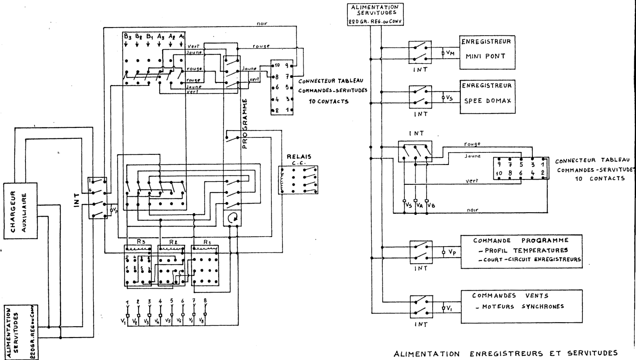
COMMANDES PROFIL TEMPERATURES EAU
