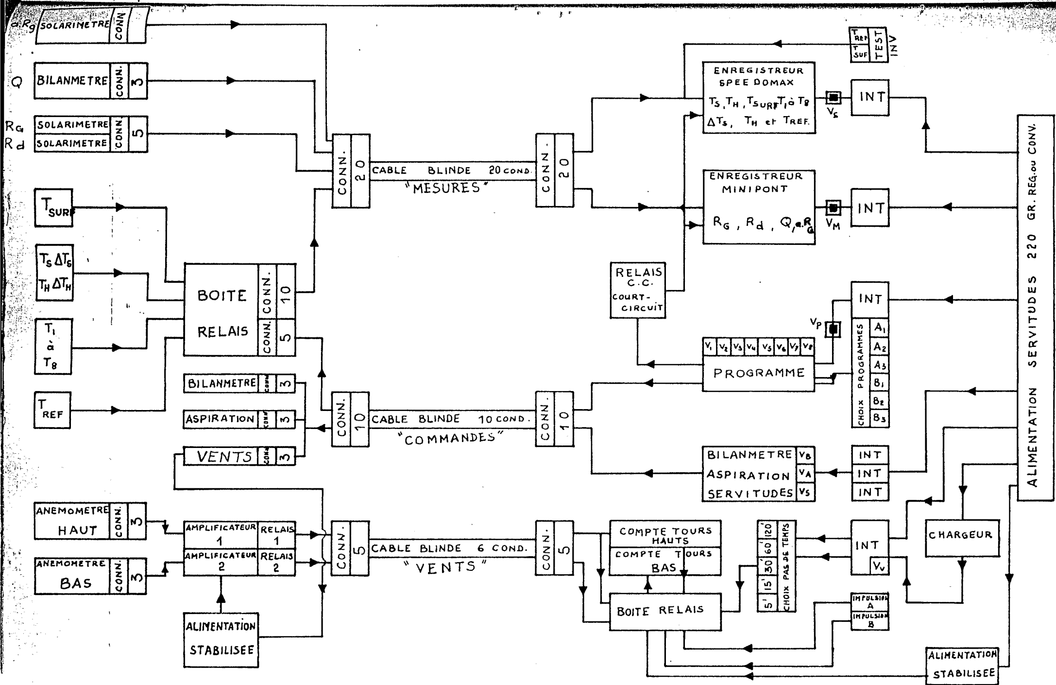
SCHEMA DU DISPOSITIF DE MESURE ET DE COMMANDE
