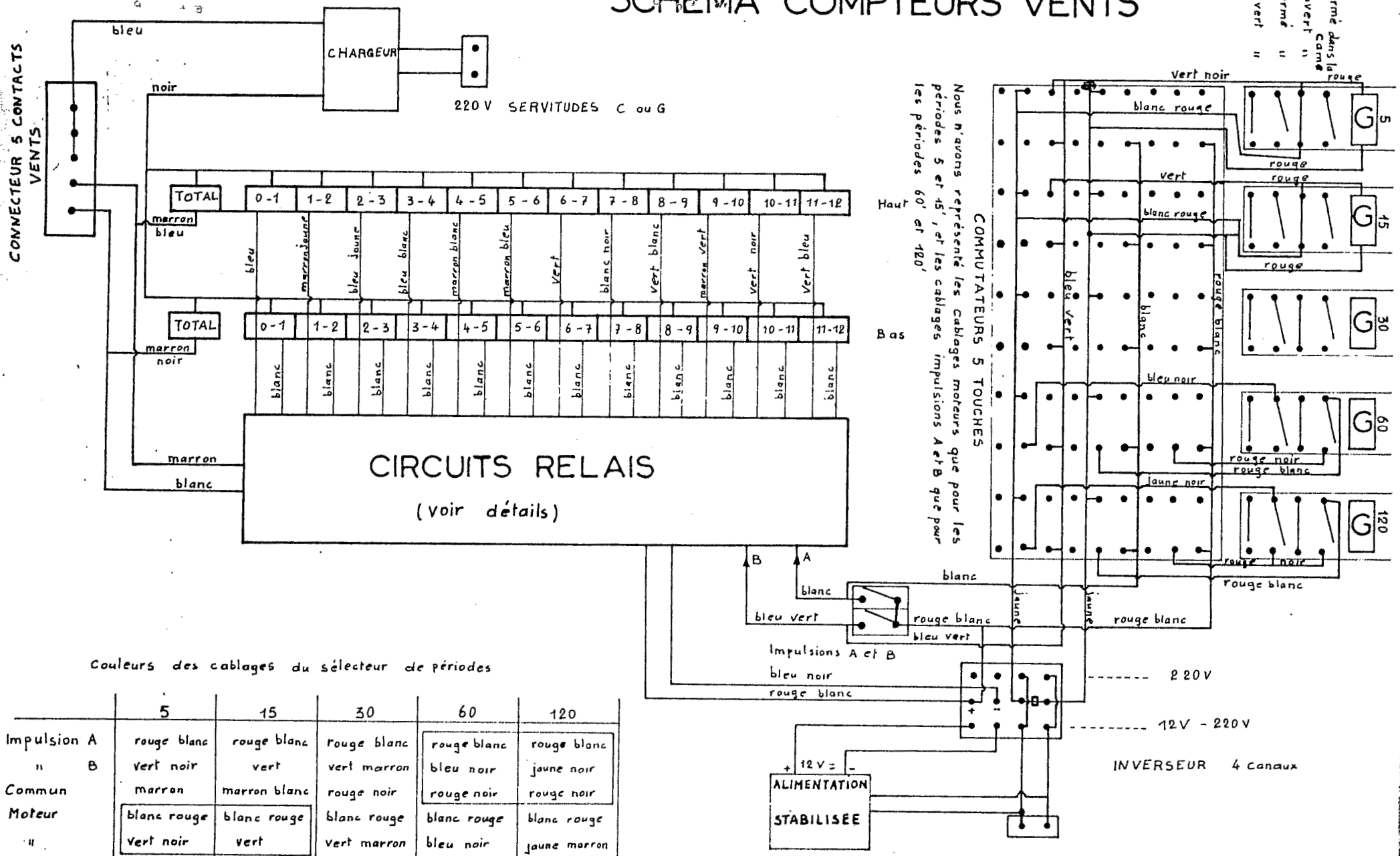
Les cablages encadrés sont représentés sur le schéma suivant
