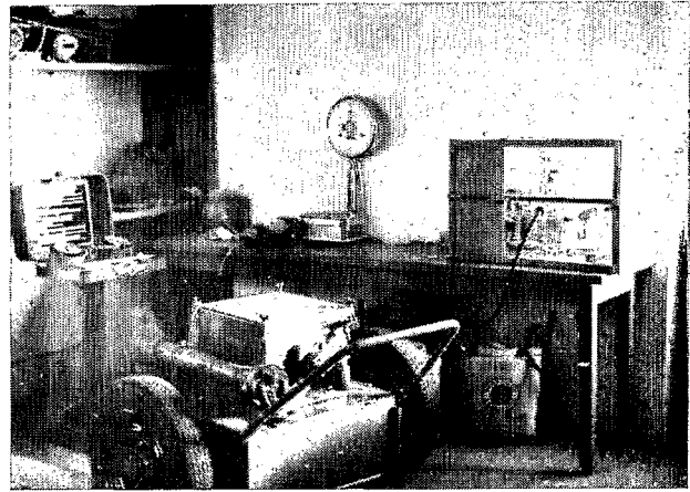
D. M. A. G. R. : Hall d'essais (banc Muller. dynamomètre Amsler...)
