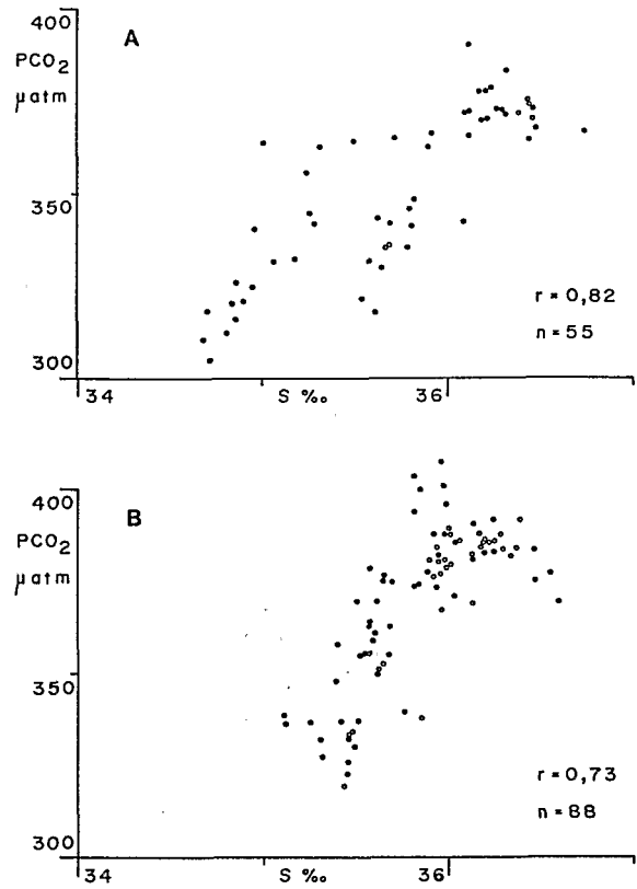
Figure 7 Variation de la pression partielle de CO 2 océanique PCO 2 (μatm) en fonction de la salinité S à la surface de la mer entre 4°W et 35°W, 5°S et 14°N, en janvier (A) et en juillet (B) 1983. Surface seawater CO 2 partial pressure PCO 2 (μatm) versus sea surface salinity S between 4°W and 35°W, 5°S and 14°N, in January (A) and in July (B) 1983.
