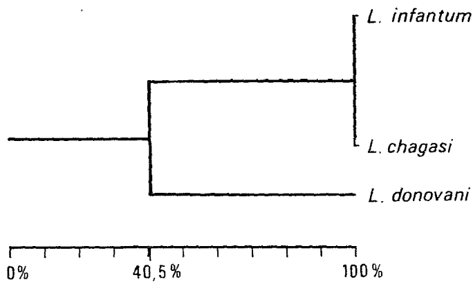
Figure 2 — Relation phylogénique supposée entre espèces du complexe Leishmania donovani , basée sur le degré de similitude protéique (% de bandes communes).
