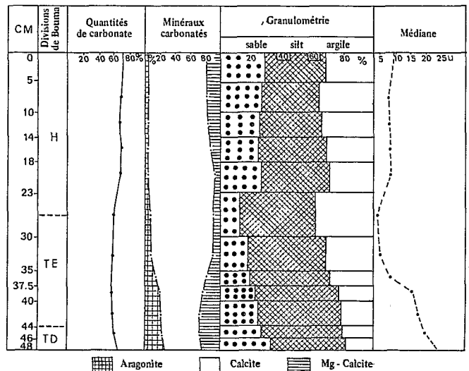
Figure 7 Variation de quelques paramètres granulométriques et minéralogiques le long de la séquence S8 (carotte 97) TD, TE : turbidite; H : hémipélagite. Variation of some granulometric and mineralogical parameters through the S8 sequence (core 97).
