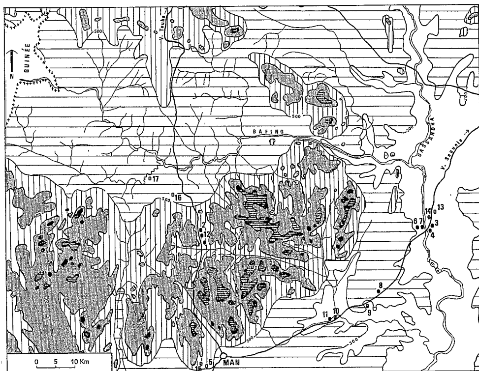
Fig. 2. — Esquisse topographique.
