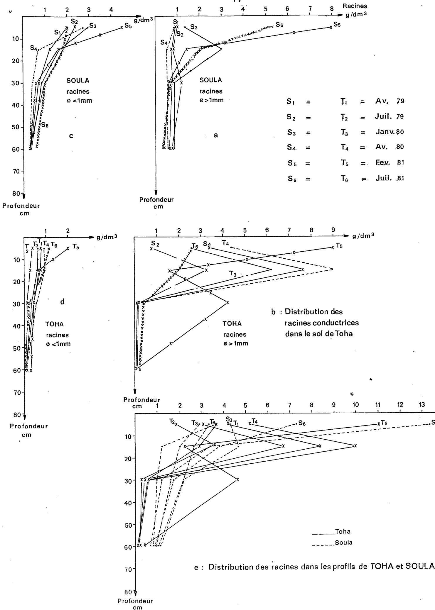
FIG. 5 : DISTRIBUTION VERTICALE DES TAUX DE RACINES DANS LES SOLS DE SOULA ET DE CEUX DE TOHA
