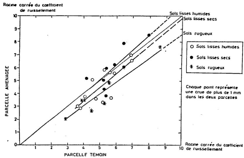
Fig. 8 COMPARAISON DES COEFFICIENTS DE RUISSELLEMENT ENTRE LA PARCELLE AMENAGEE ET LA PARCELLE TEMOIN POUR UN AMENAGEMENT CLOISONNE ET SANS IMPLUVIUM
