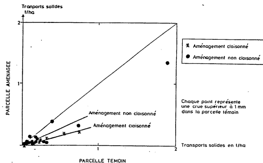
Fig. 5 COMPARAISON DES EROSIONS ENTRE LA PARCELLE AMENAGEE ET LA PARCELLE TEMOIN
