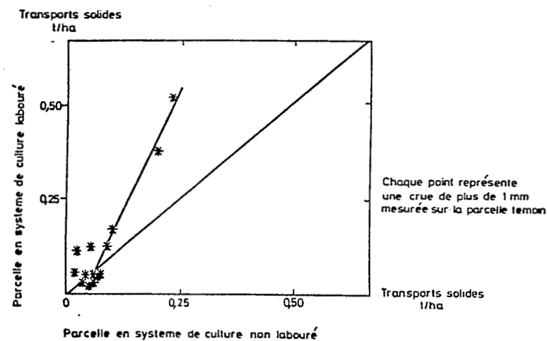
Fig. 6 COMPARAISON DES EROSIONS SUR LA PARCELLE EN SYSTEME DE CULTURE LABOURE ET EN SYSTEME DE CULTURE SANS LABOUR
