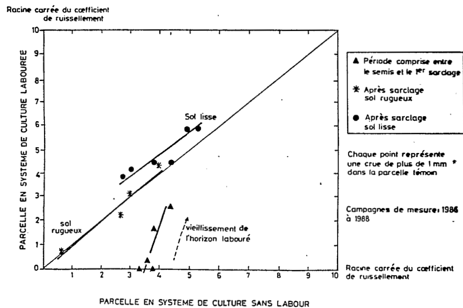
Fig. 4 COMPARAISON DES COEFFICIENTS DE RUISSELEMENT DE DEUX PARCELLES IDENTIQUES SOUMISES A DEUX PARCELLES SYSTEMES DE CULTURES DIFFERENTES
