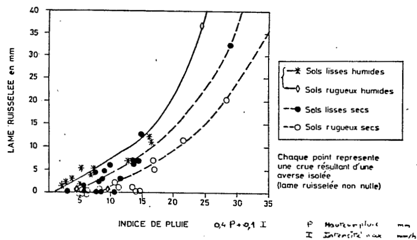
Fig. 4 COMPARAISON DES COEFFICIENTS DE RUISSELEMENT DE DEUX PARCELLES IDENTIQUES SOUMISES A DEUX PARCELLES SYSTEMES DE CULTURES DIFFERENTES
