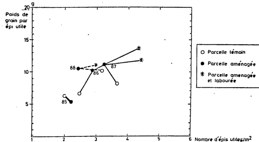
Fig. 10 CROISEMENT DES VARIABLES POIDS DE GRAIN PAR EPI ET NOMBRE D'EPIS UTILES/m² SUR LES STATIONS DE LA MOITIE INFERIEURE DES PARCELLES
