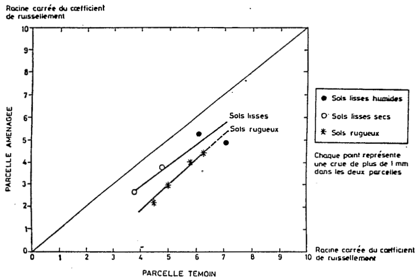
Fig. 8 COMPARAISON DES COEFFICIENTS DE RUISSELLEMENT ENTRE LA PARCELLE AMENAGEE ET LA PARCELLE TEMOIN POUR UN AMENAGEMENT CLOISONNE ET SANS IMPLUVIUM
