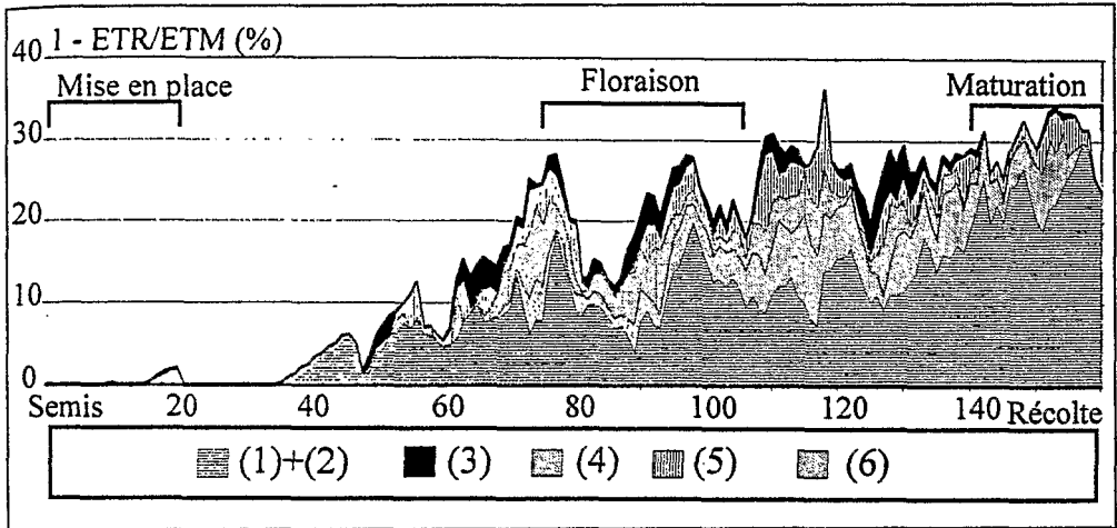
Figure 4 - Evolution des déficits hydriques simulés du maïs (cycle de 160 jours) au cours de la période de culture (moyennes pour l'ensemble des parcelles cultivées). La courbe enveloppe représente le déficit total. Les nombres de la légende correspondent avec ceux donnés dans le tableau 2.
