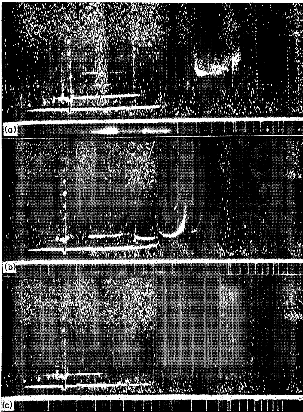
FIG. 1. TYPICAL IONOGRAMS: a) F1-lacuna b) F2-lacuna c) total lacuna.
