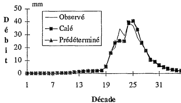
Figure n° 7 La Tiemba à Dioulatiedougou, 1981. Hydrogrammes observés, calés et prédéterminés. Modèle GR3.
