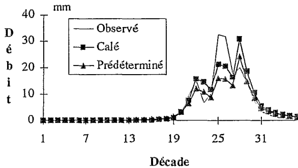
Figure n° 8 La Tiemba à Lille, 1984. Hydrogrammes observés, calés et prédéterminés. Modèle GR3.
