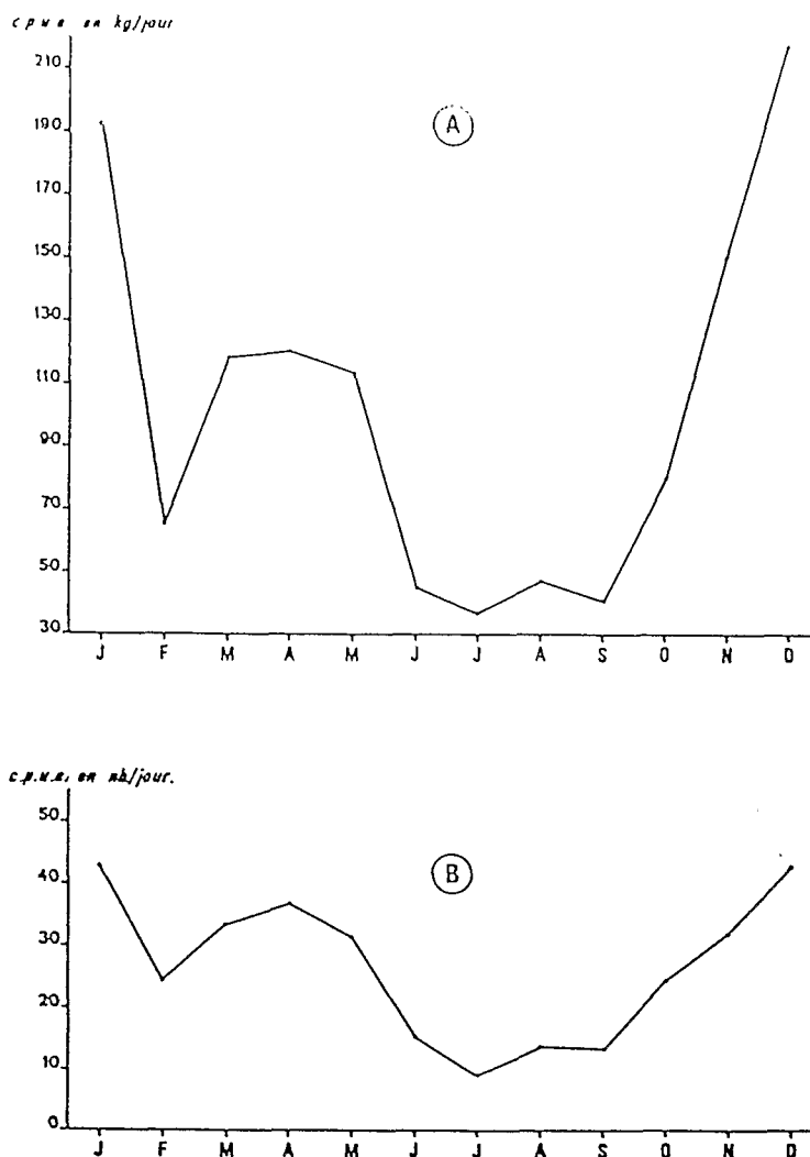
Fig. 6 : PRISE TOTALE-VARIATIONS MENSUELLES DES RENDEMENTS EN POIDS (A) ET EN NOMBRE (B).
