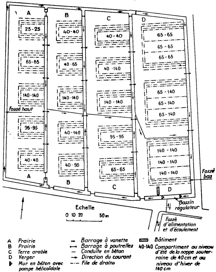
Fig. 1. — Aménagement d'un champ d'essai pour l'étude du niveau de la nappe (ferme De Vlierd, Pays-Bas).
