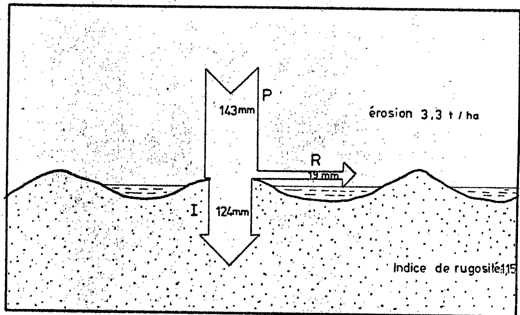
b) Labour molteux seul : rugosité forte forte détention superficielle
