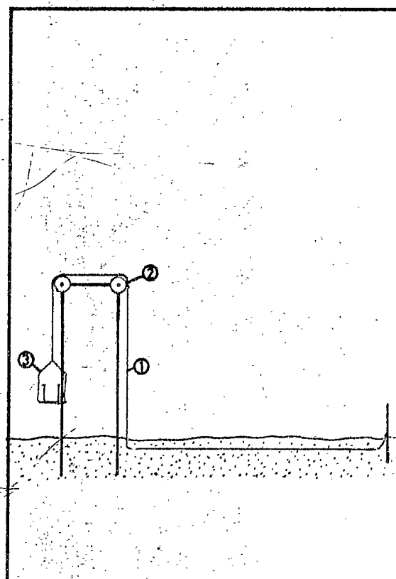
b) Méthode de fil de pêche enterré (d'après Bennet et al. 1964)
