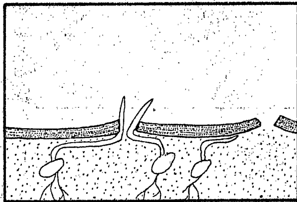
b) Les plantules contournent la croûte
