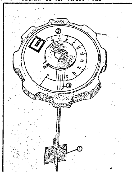
d) Scissomètre (modèle Pilcon)
