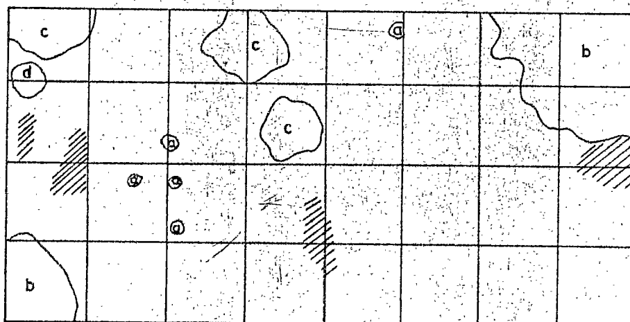
b) Carte des états de surface élémentaires
