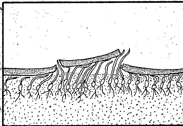
c) Les plantules soulèvent des éléments de la croûte
