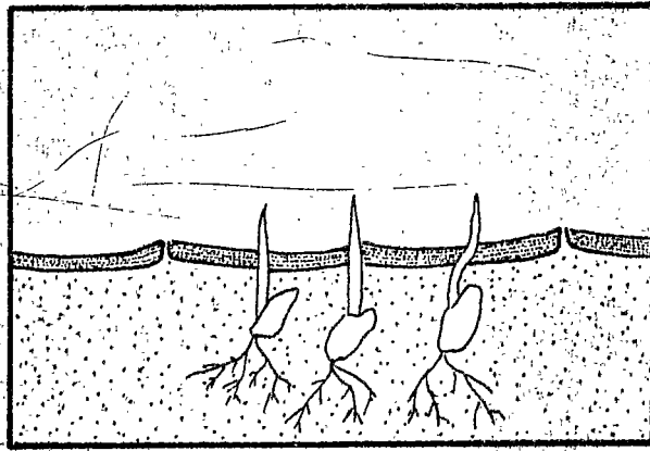
a) Les plantules percent la croûte
